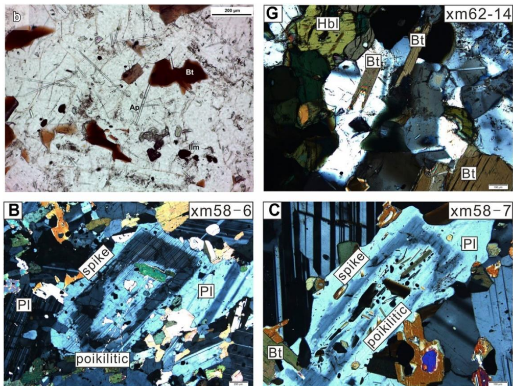
Рисунок 2.3. Примеры неравновесных петрографических структур в гибридных породах, формирующихся при взаимодействии контрастных по составу магм. b – игольчатый апатит (Clemens, Bezuidenhout, 2014); G – лезвиеподобный биотит; B , C – пойкилитовая структура, неоднородная зональность и узкие анортитовые зоны (spike) в низкокальциевых зонах плагиоклазов (Ma et al., 2021).
