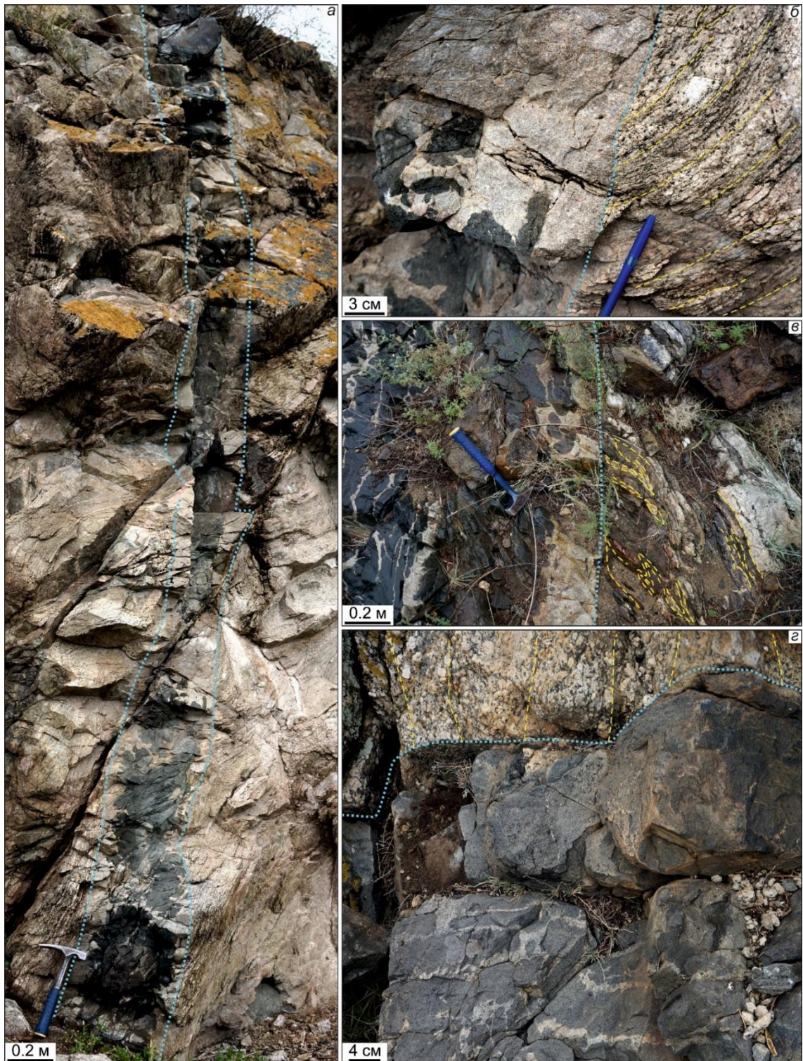
Рисунок 4.3. Внутреннее строение комбинированных даек участков Баянкол ( а, б ), РЛС ( в ), Матут ( г ). а – субвертикальная дайка с центральной мафической и краевой салической частью; б – секущие контакты дайки и мигматитов эрзинского комплекса; в – округлые нодулы диоритов в краевой части дайки; г – секущие контакты дайки и крупнопорфировых гранитов. Голубым пунктиром показаны контакты даек, желтым – структура вмещающих пород.
