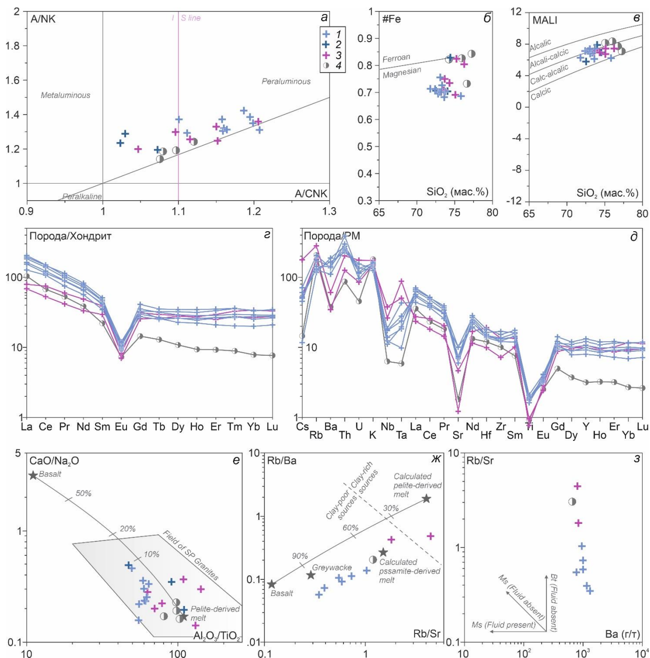
Рисунок 6.18. Особенности вещественного состава лейкогранитов комбинированных и простых даек (группа I). a – A/NK - A/CNK, I-S линия по (Chappell, White, 2001); б – \text{FeO}^{\text{tot}}/(\text{FeO}^{\text{tot}}+\text{MgO}) - \text{SiO}_2 (Frost et al., 2001); в – диаграмма с MALI (Frost et al., 2001); г – нормированные по хондриту кривые распределения редкоземельных элементов; д – нормированные по примитивной мантии мультиэлементные диаграммы (Sun, McDonough, 1989); е – диаграмма \text{CaO}/\text{Na}_2\text{O} - \text{Al}_2\text{O}_3/\text{TiO}_2 , SP – сильнопералюминиевые граниты (Sylvester, 1998); ж – диаграмма Rb/Ba - Rb/Sr (Sylvester, 1998); з – диаграмма Rb/Sr - Ba (Harris, Inger, 1992). 1 – участок Сайзырал; 2 – участки Матут, Баянкол, РЛС; 3 – простые дайки; 4 – монцолейкограниты ухадагского комплекса (Кармышева и др., 2022а).
