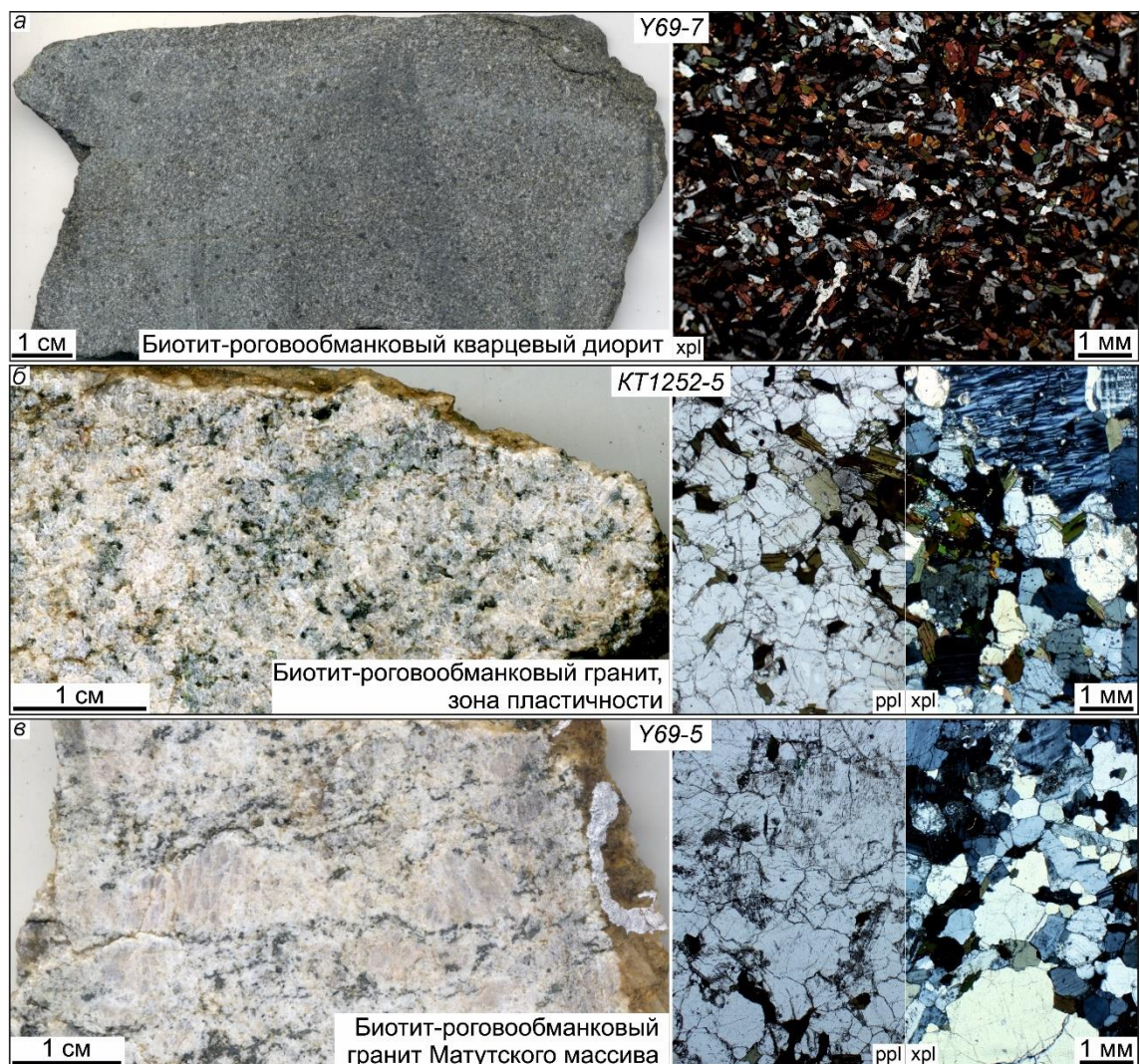
Рисунок 4.7. Петрографическая характеристика пород комбинированных даек участка Тавыт-Даг, а также вмещающих гранитов Матутского массива.
