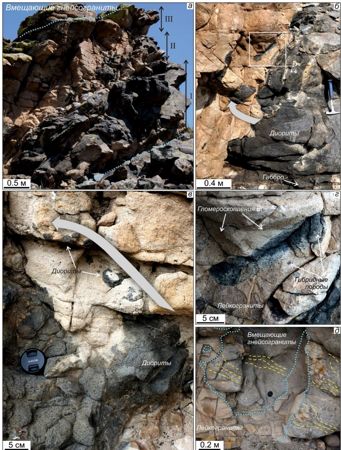
Рисунок 4.9. Строение комбинированной дайки Сайзырал. а – общий вид дайки (римскими цифрами обозначены нижняя, средняя и верхняя части дайки); б , в – структуры отрыва в средней части дайки; г – переходные породы в средней части дайки; д – секущий контакт дайки с вмещающими породами. Голубым пунктиром показаны контакты пород дайки и вмещающих гнейсогранитов, желтым пунктиром – гнейсовидная структура вмещающих пород. Серыми стрелками показано направление отрыва фрагментов диоритов.
