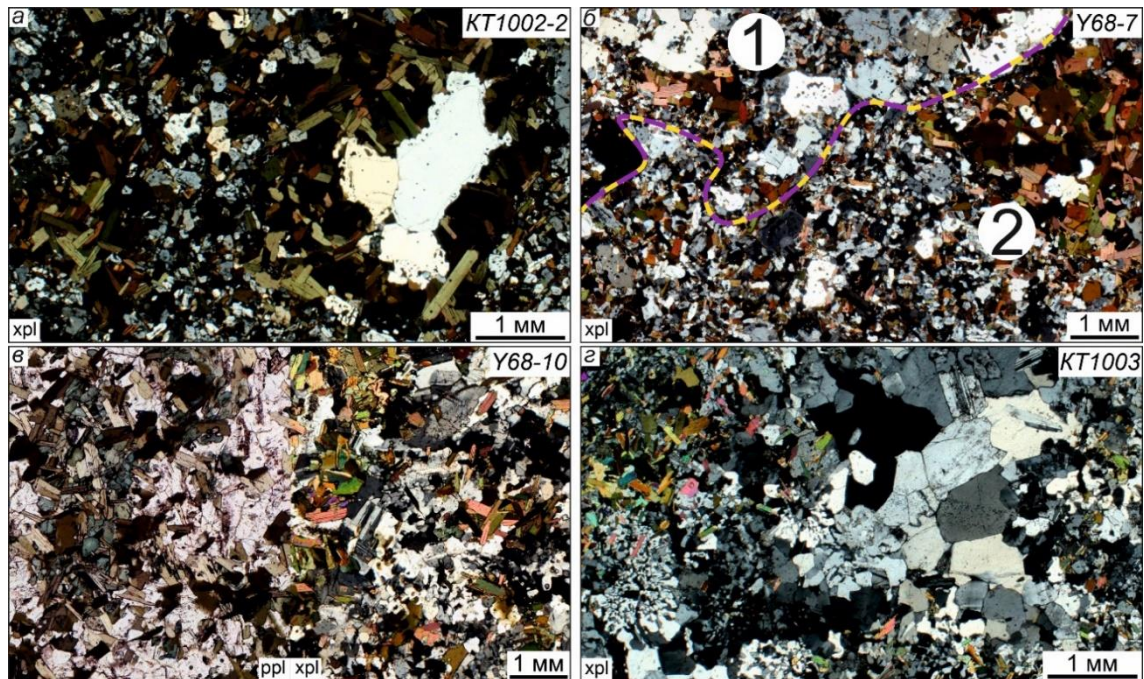
Рисунок 4.11. Взаимоотношения контрастных пород комбинированной дайки Сайзырал. а – гломероскопления биотита в зоне промежуточного состава; б – контакт гранита (1) и гибридной породы (2), пунктирной линией показан контакт; в – гибридная порода из промежуточной зоны; г – рекристаллизованный гранит.
