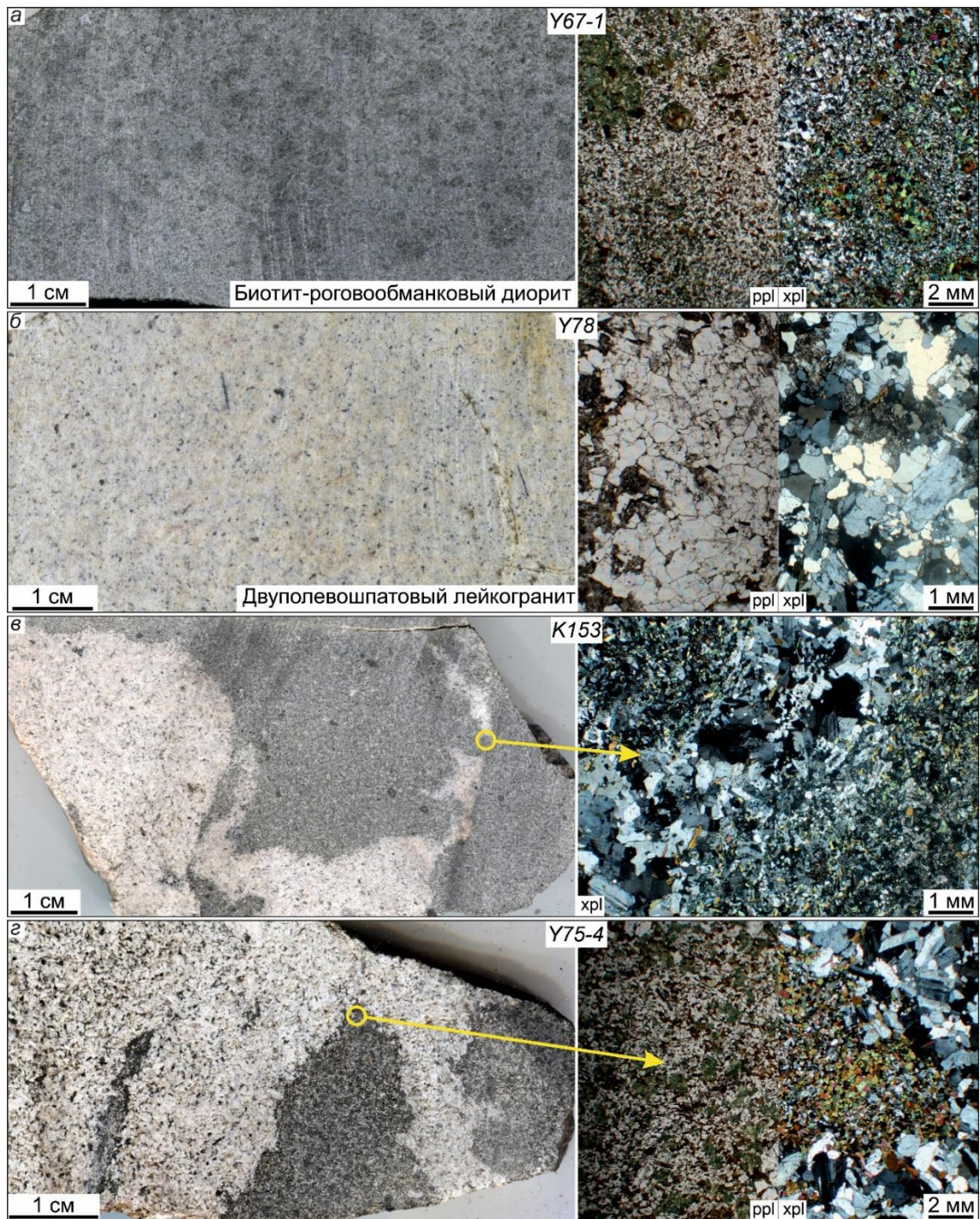
Рисунок 4.4. Петрография и взаимоотношения контрастных пород комбинированных даек участков Баянкол, Матут, РЛС. в – рекристаллизация кварца в тонком гранитном «прожилке»; г – четкие фестончатые контакты контрастных пород без промежуточных зон и закалки.
