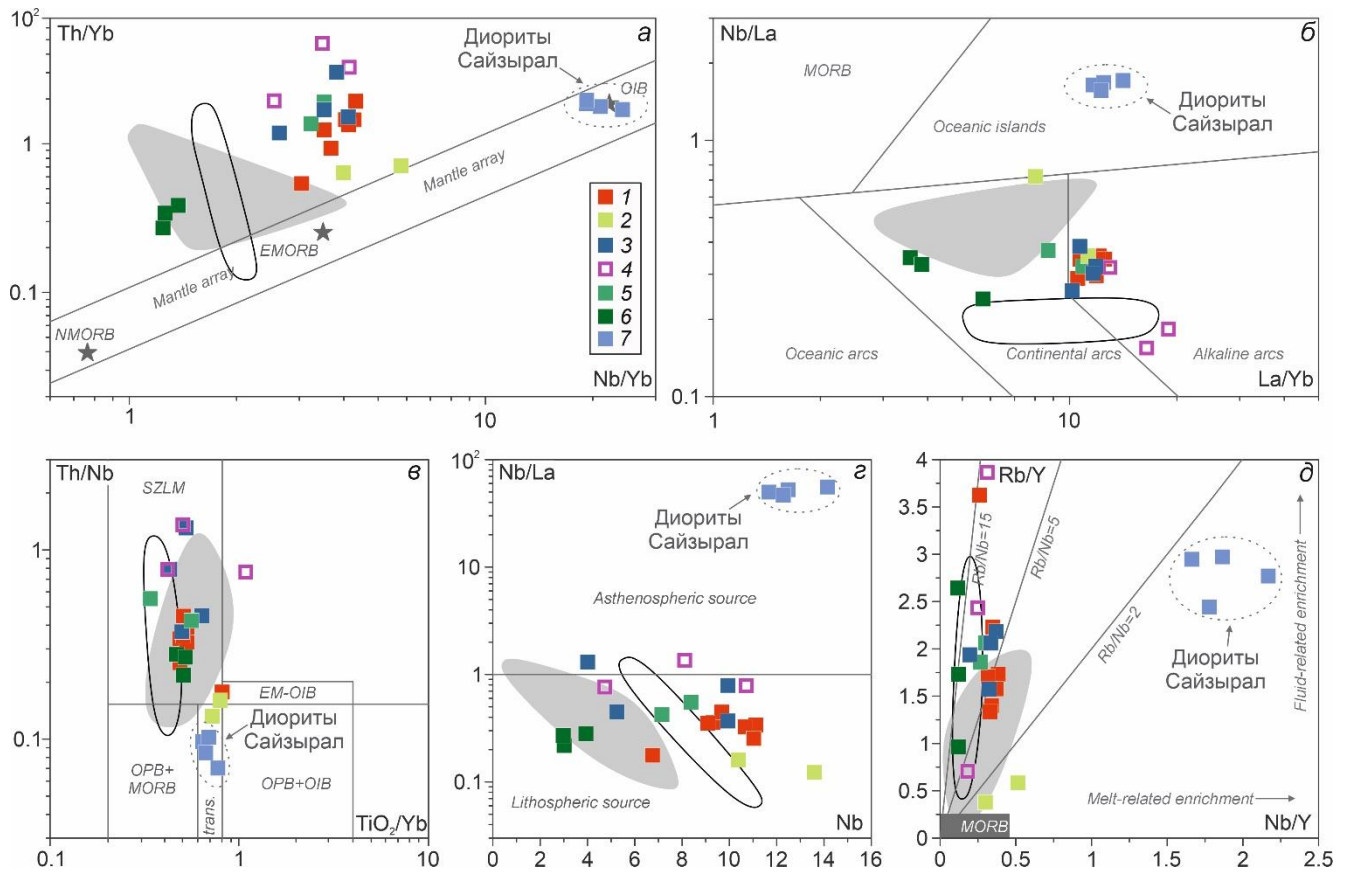
Рисунок 6.17. Дискриминационные диаграммы для мафических пород комбинированных, синплутонических и простых даек. a – Th/Yb - Nb/Yb (Pearce, 2008); б – Nb/La - La/Yb (Hollocher, 2012); в – Th/Nb - TiO 2 /Yb (Pearce et al., 2021); г – Nb/La - Nb (Smith et al., 1999); д – Rb/Y - Nb/Y (Temel et al., 1998). MORB – mid-ocean ridge basalt, OIB – oceanic island basalt, EM-OIB – enriched mantle-rich OIB, OPB – oceanic plateau basalt, SZLM – subduction-modified lithospheric mantle. 1 – дайка Тавыт-Даг, 2 – габбро дайки Сайзырал, 3 – дайки участков Матут, Баянкол, РЛС, 4 – простые дайки, 5 – дайки Стрелка, 6 – дайки Восточный, 7 – диориты дайки Сайзырал. Серым полем показаны составы габброноритов Баянкольского массива, черным контуром – составы монцодиоритов Эрзинского массива по (Shelepaev et al., 2018).
