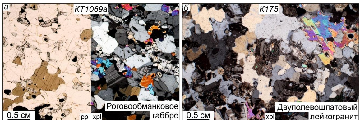
Рисунок 4.2. Петрографическая характеристика пород простых базитовых (а) и лейкогранитных даек (б).
