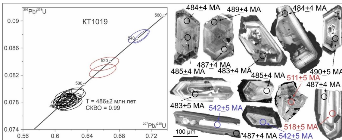
Рисунок 5.3. Диаграммы с конкордией и катодоллюминесцентные изображения цирконов из простых лейкогранитных даек (Karmysheva et al., 2021).
