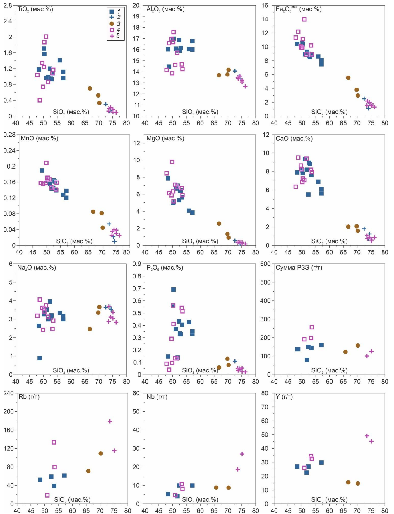
Рисунок 6.2. Содержания пороодообразующих (мас. %) и редких (г/т) элементов по отношению к \text{SiO}_2 для пород комбинированных даек участков Баянкол, Матут и РЛС, а также простых базитовых и лейкогранитных даек. 1-3 – комбинированные дайки: 1 – габбро и диориты, 2 – лейкограниты, 3 – граниты; 4,5 – простые дайки: 4 – габбро, 5 – лейкограниты.
