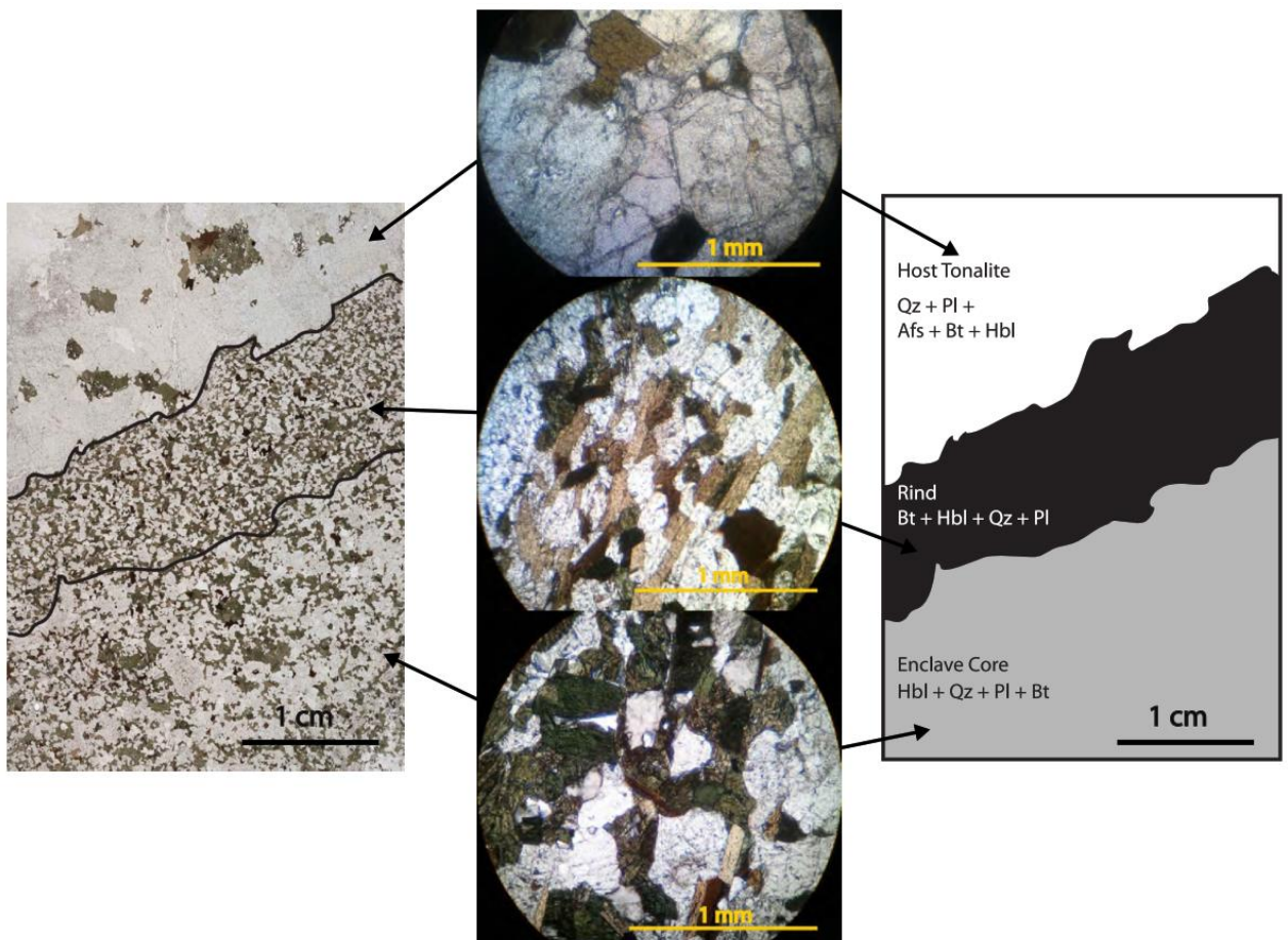
Рисунок 2.4. Петрографические особенности краевых зон магматических включений, насыщенных биотитом (Farner et al., 2014).
