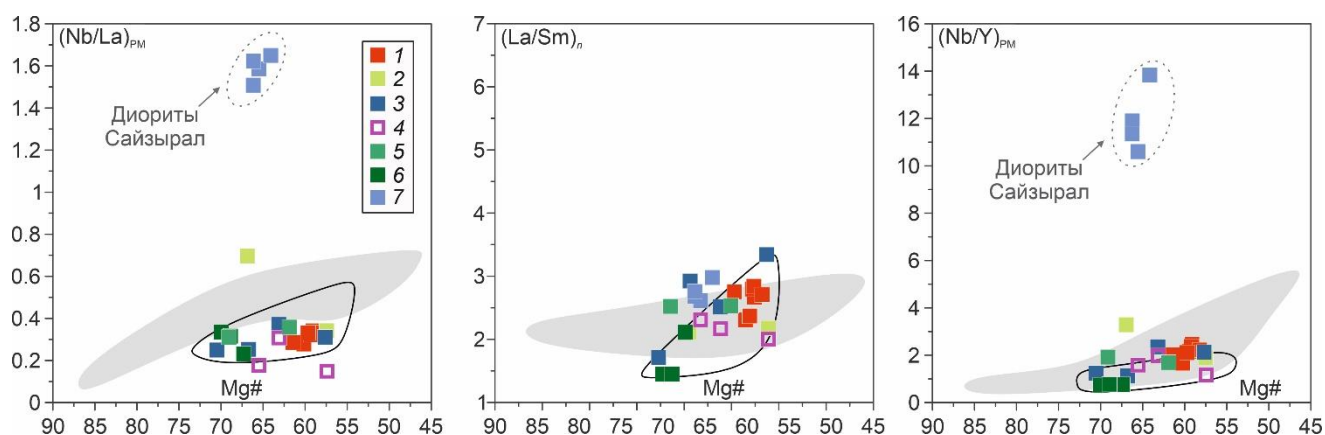
Рисунок 6.15. Вариации содержания редких (г/г) элементов в мафических породах комбинированных, синплутонических и простых даек относительно \text{Mg\#} . 1 – дайка Тавыт-Даг, 2 – габбро дайки Сайзырал, 3 – дайки участков Матут, Баянкол, РЛС, 4 – простые дайки, 5 – дайки Стрелка, 6 – дайки Восточный, 7 – диориты дайки Сайзырал. Серым полем показаны составы габброноритов Баянкольского массива, черным контуром – составы монцодиоритов Эрзинского массива по (Shelepaev et al., 2018).
