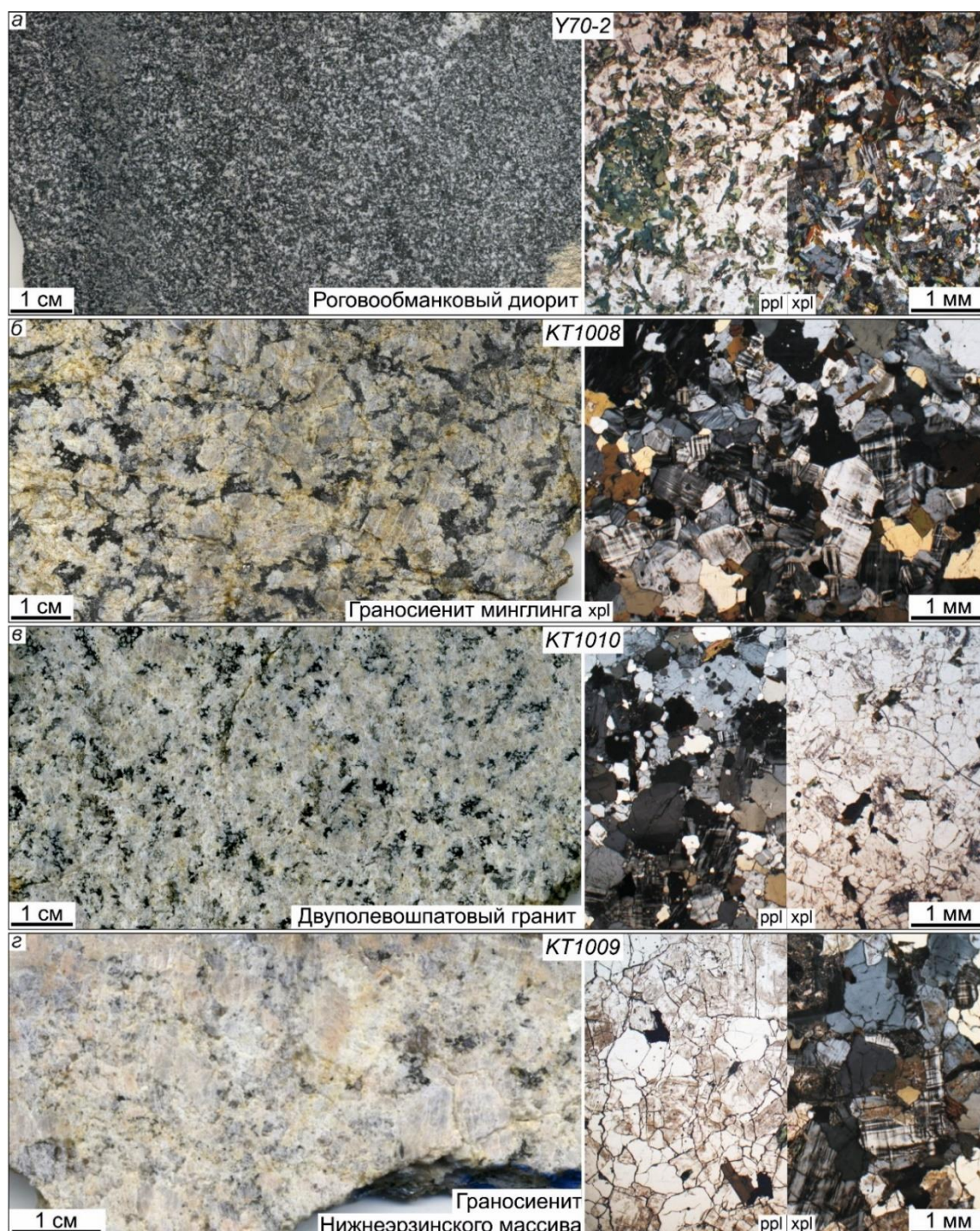
Рисунок 4.14. Петрография пород синплутонических даек участка Стрелка.
