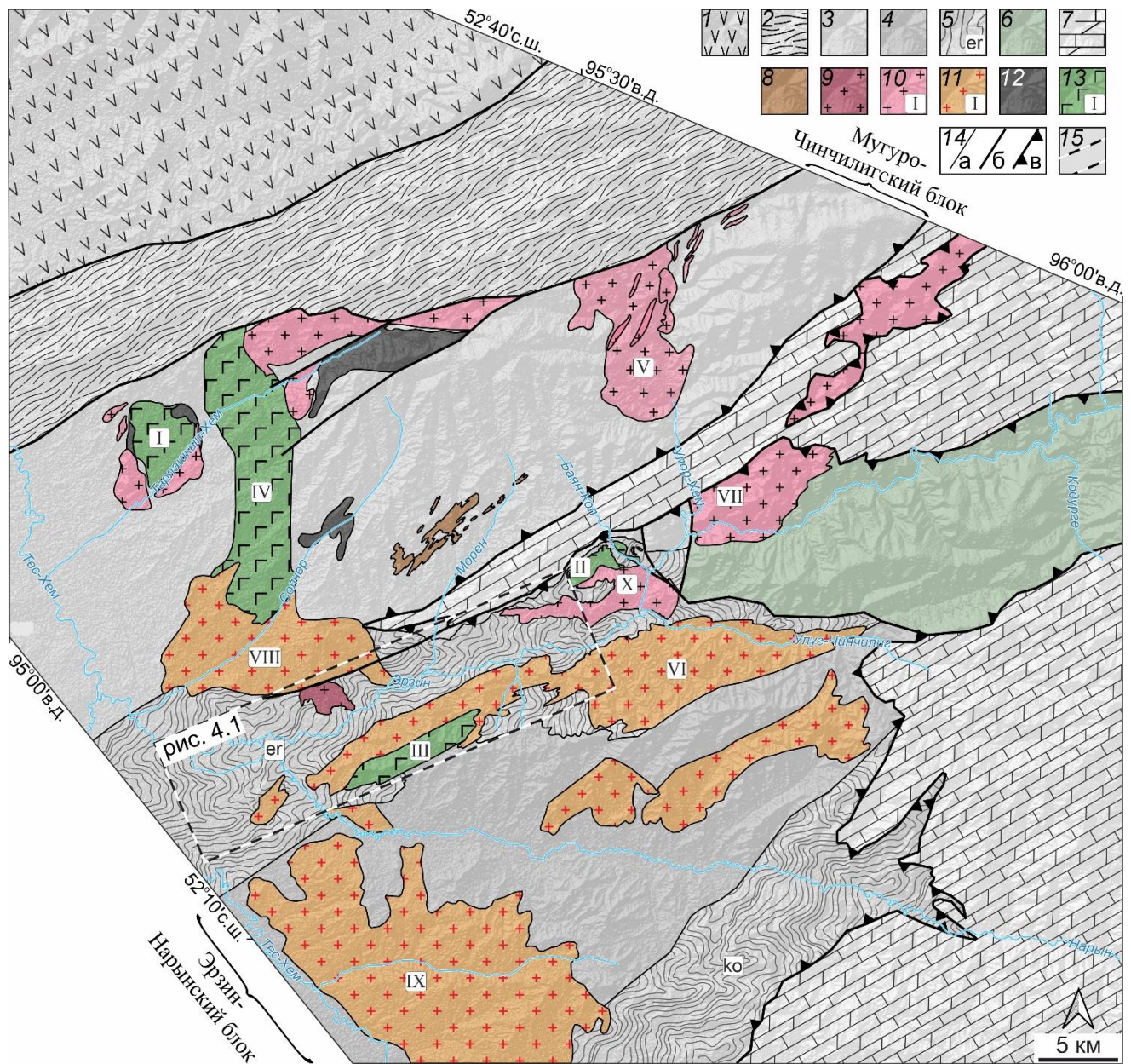
Рисунок 3.2. Схема геологического строения Западного Сангилена по (Владимиров и др., 2005, 2017; Кармышева и др., 2022a). 1 – Таннуольская островная дуга; 2 – офиолиты Агардагской зоны; 3-6 – метаморфические комплексы: 3 – моренский, 4 – тесхемский, 5 – эрзинский, 6 – чинчиллигский; 7 – терригенно-карбонатные породы сангиленской серии; 8-11 – гранитоидные массивы: 8 – ортоадырского комплекса, 9 – Матутский гнейсогранитный I-типа, 10 – прочие массивы I-типа; 11 – ухадагского комплекса (А-тип); 12 – гипербазитовые массивы; 13 – габбро-монцодиоритовые массивы; 14 – геологические границы: а – магматических и метаморфических комплексов, б – крутопадающие разломы, в – надвиги; 15 – область исследований. Буквенные обозначения отвечают распространению пород эрзинского комплекса в пределах Эрзинской (er) и Кокмолгаргинской (ко) тектонических зон. Римские цифры обозначают магматические массивы: I – Правотарлашкинский, II – Баянкольский габбро-монцодиоритовый, III – Эрзинский, IV – Башкымугурский, V – Улорский, VI – Нижнеэрзинский, VII – Нижнеулорский, VIII – Ухадагский, IX – Тесхемский, X – Баянкольский гранодиоритовый.
