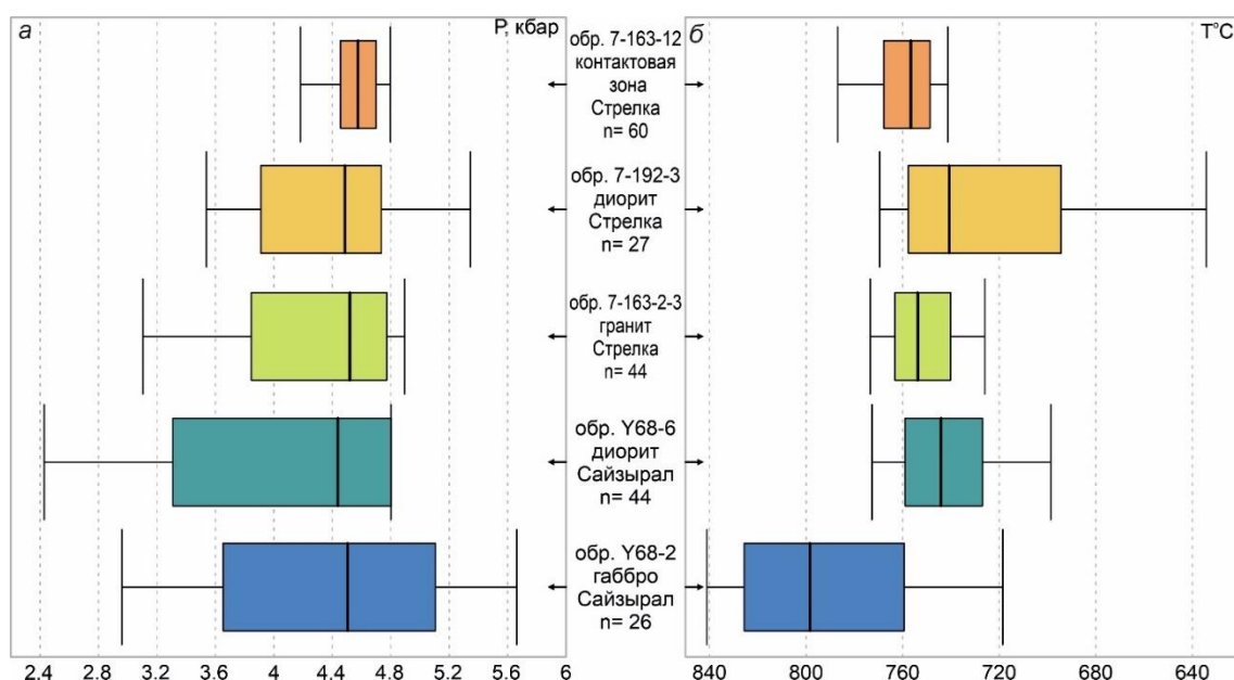
Рисунок 4.19. Обобщенные результаты вычислений давления и температур кристаллизации пород минглинг даек участков Сайзырал и Стрелка с использованием геотермобарометров (Holland, Blundy, 1994; Putirka, 2016; Rudolphi, Renzulli, 2012).
