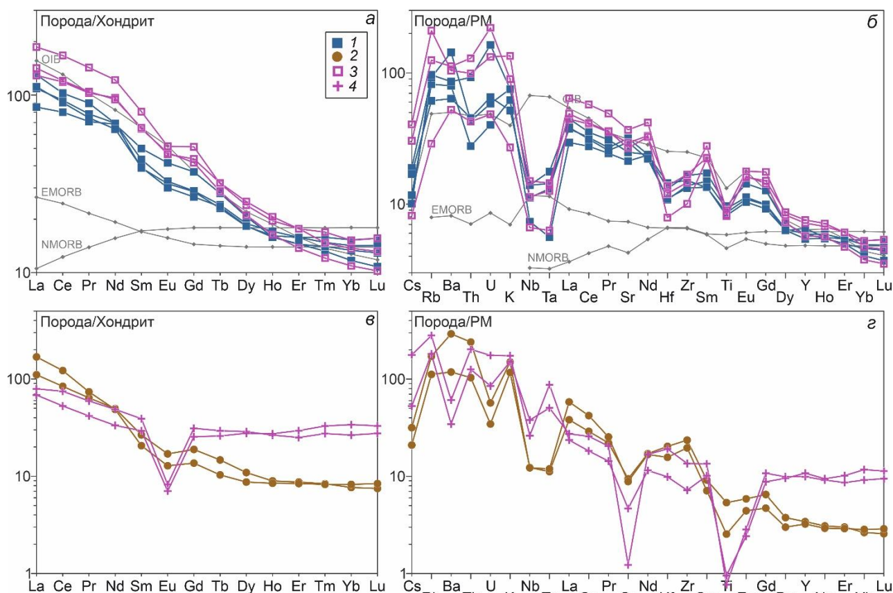
Рисунок 6.4. Нормированные по хондриту кривые распределения редкоземельных элементов (а, в) и нормированные по примитивной мантии мультиэлементные диаграммы (б, з) для пород комбинированных даек участков Баянкол, Магут и РЛС, а также простых базитовых и лейкогранитных даек. Данные для хондрита, примитивной мантии, MORB и OIB по (Sun, McDonough, 1989). 1,2 – комбинированные дайки: 1 – габбро и диориты, 2 – граниты; 3,4 – простые дайки: 3 – габбро, 4 – лейкограниты.
