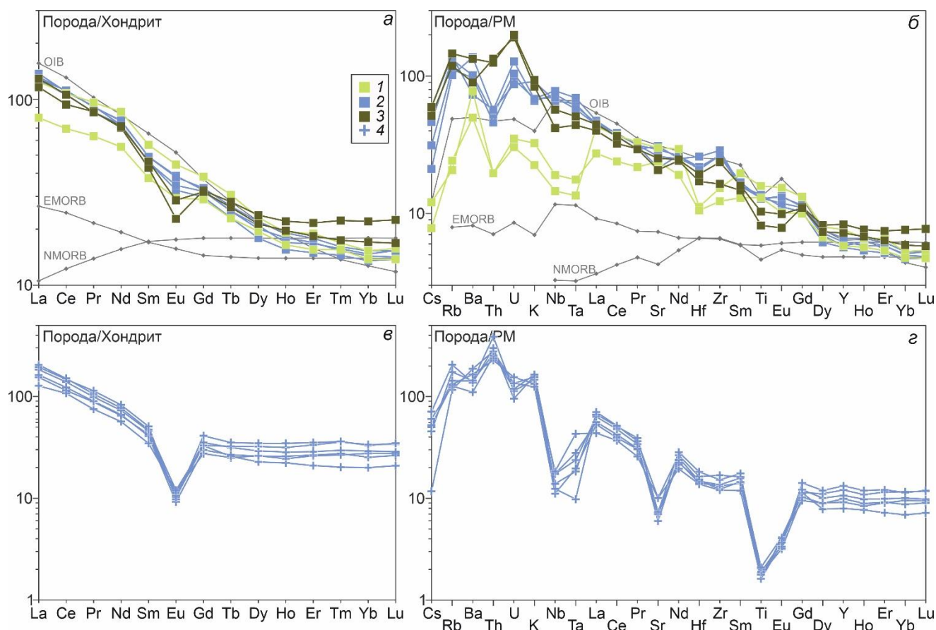
Рисунок 6.9. Нормированные по хондриту кривые распределения редкоземельных элементов (а, в) и нормированные по примитивной мантии мультиэлементные диаграммы (б, з) для пород комбинированной дайки участка Сайзырал. Данные для хондрита, примитивной мантии, MORB и OIB по (Sun, McDonough, 1989). 1 – габбро, 2 – диориты, 3 – породы переходных зон, 4 – лейкограниты.
