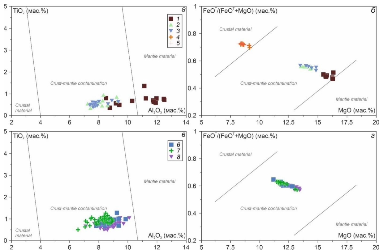
Рисунок 6.24. Генетические диаграммы для амфиболов (а, в, Jiang, An, 1984) и биотитов (б, з, Guo et al., 2017) минглинг даек участков Сайзырал (а, б) и Стрелка (в, з). 1-5 минералы пород комбинированной дайки Сайзырал: 1 – габбро, 2 – диорит, 3 – породы переходных зон, 4 – лейкогранит (основная масса), 5 – лейкогранит (гломероскопления). 6-8 минералы пород синплутонических даек Стрелка: 1 – диорит, 2 – гранит, 3 – породы переходных зон.
