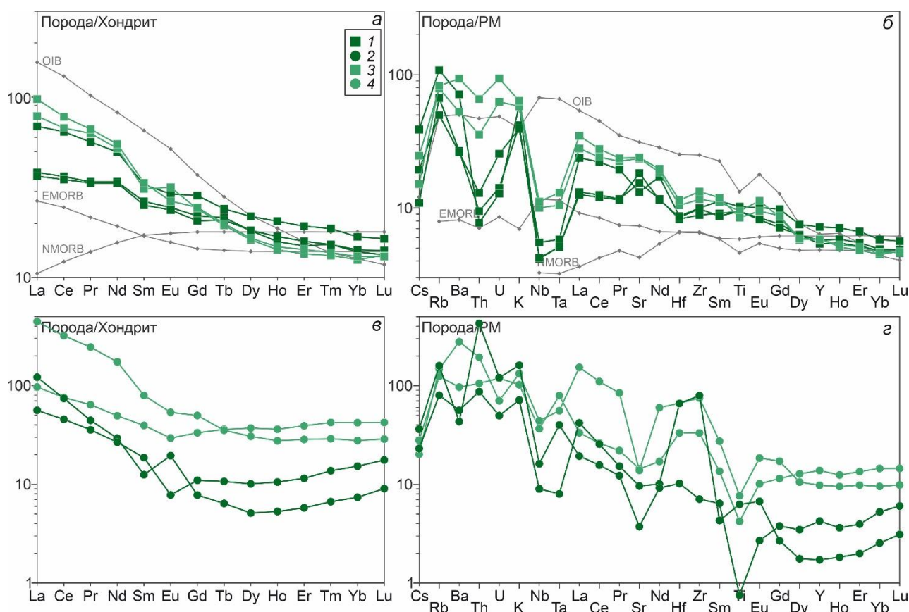
Рисунок 6.13. Нормированные по хондриту кривые распределения редкоземельных элементов (а, в) и нормированные по примитивной мантии мультиэлементные диаграммы (б, з) для пород синплутонических даек участков Стрелка и Восточный. Данные для хондрита, примитивной мантии, MORB и OIB по (Sun, McDonough, 1989). 1,2 – Восточный: 1 – габбро и диориты, 2 – гранитоиды; 3,4 – Стрелка: 3 – габбро и диориты, 4 – гранитоиды.
