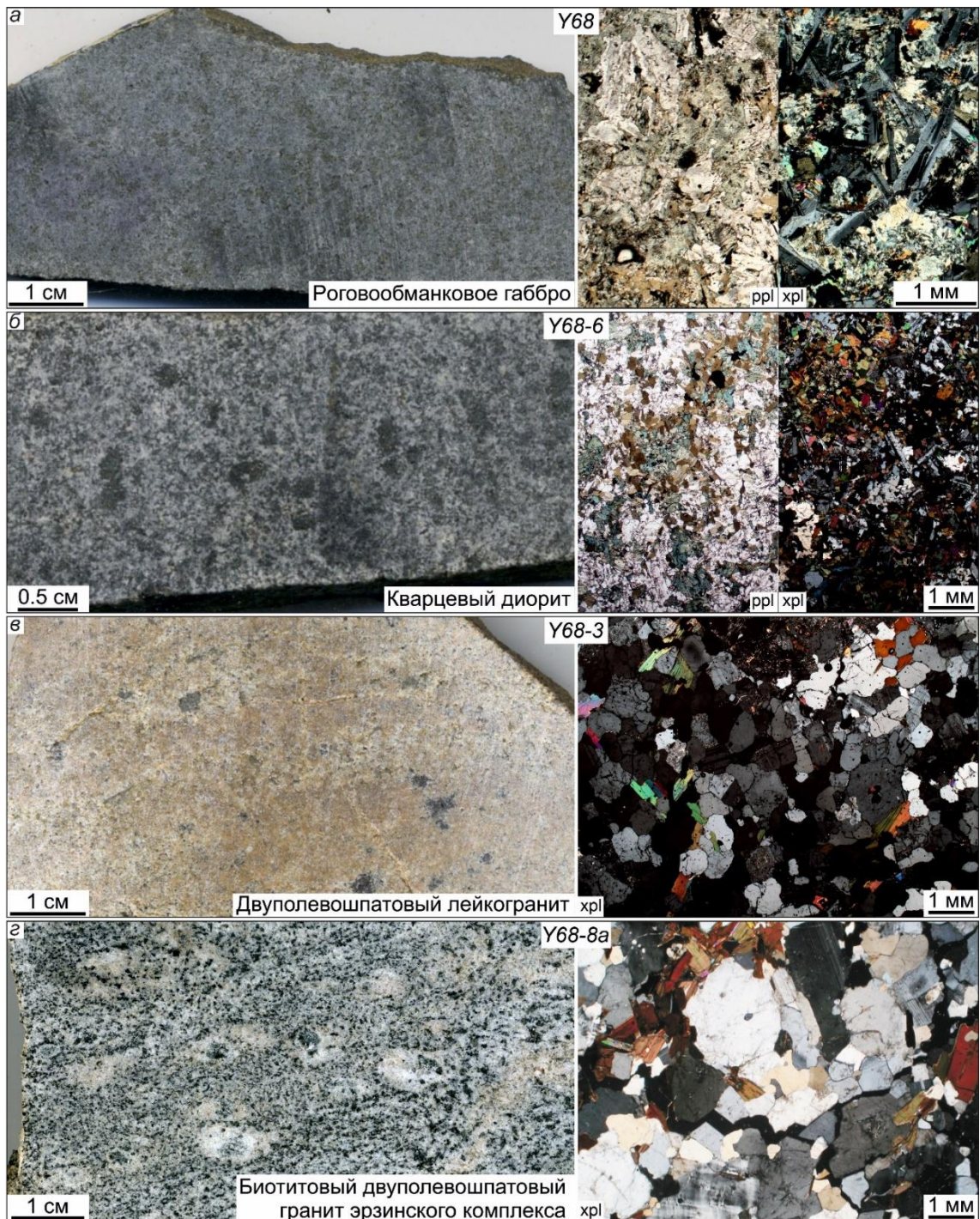
Рисунок 4.10. Петрографическая характеристика пород комбинированной дайки участка Сайзырал, а также вмещающих гранитов эрзинского комплекса.
