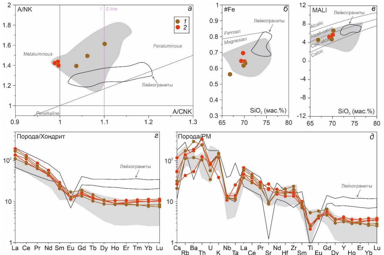
Рисунок 6.21. Особенности вещественного состава гранитов комбинированных даек. а – A/NK - A/CNK, I-S линия по (Chappell, White, 2001); б – FeO^{tot}/(FeO^{tot}+MgO) - SiO_2 (Frost et al., 2001); в – диаграмма с MALI (Frost et al., 2001); з – нормированные по хондриту кривые распределения редкоземельных элементов; д – нормированные по примитивной мантии мультиэлементные диаграммы (Sun, McDonough, 1989). 1 – биотит-роговообманковые граниты комбинированной дайки участка Тавыт-Даг; 2 – биотитовые граниты комбинированных даек участков Матут, Баянкол и РЛС. Серым полем показаны параавтохтонные граниты эрзинского мигматит-гранитного комплекса (Кармышева и др., 2017). Черным контуром показаны лейкограниты комбинированных и простых даек (группа I).
