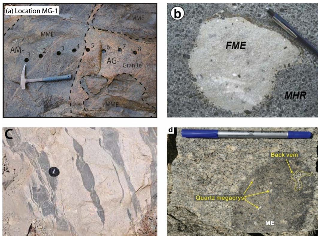
Рисунок 2.7. Фотографии обнажений магматических микрогранулярных включений. a – крупные (до 1 м) мафические включения диоритов (ММЕ) эллипсовидной формы в порфировидных гранитах (Kim et al., 2014); b – фельзитическое включение монцосиенитов (FME) в габбро (MHR) (Temizel, 2014); c – ММЕ хрупко-пластично деформированные (Farner et al., 2014); d – ММЕ с признаками смешения на мезоуровне (Lei et al., 2021).
