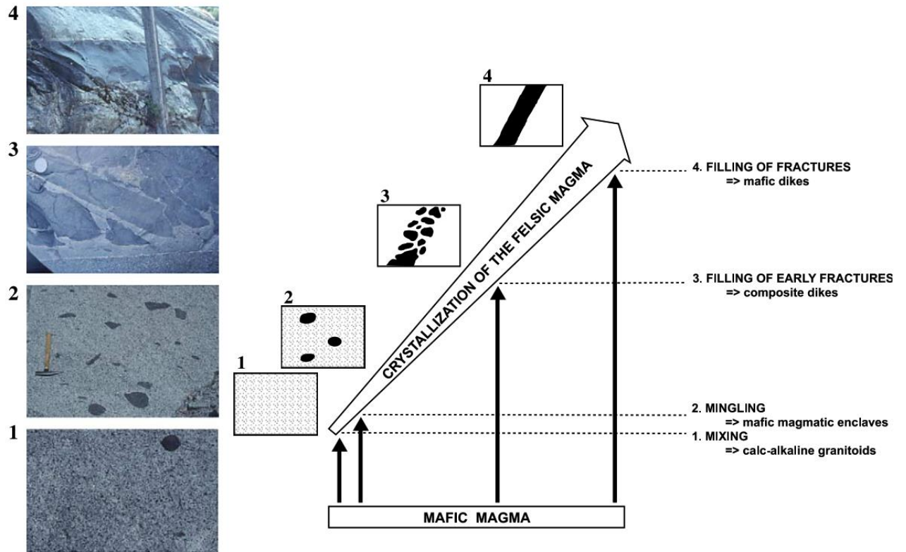
Рисунок 2.9. Принципиальная схема формирования различных типов мафических интрузий в зависимости от степени кристалличности вмещающих гранитоидов (плутон Dinkey Creek, Калифорния) (Barbarin, 2005).
