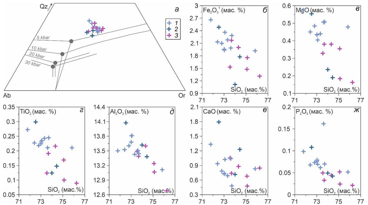
Рисунок 6.19. Особенности петрохимического состава лейкогранитов комбинированных даек (группа I). a – диаграмма Qz-Ab-Or, круги и линии показывают точки эвтектики и котектические кривые для гаплогранитной системы при a_{H_2O} = 1 и различных давлениях (модифицировано Bartoli et al., 2016 по Holtz et al., 1992); б-ж – вариации содержаний петрогенных компонентов относительно SiO_2 (мас. %). 1 – участок Сайзырал; 2 – участки Матут, Баянкол, РЛС; 3 – простые дайки.
