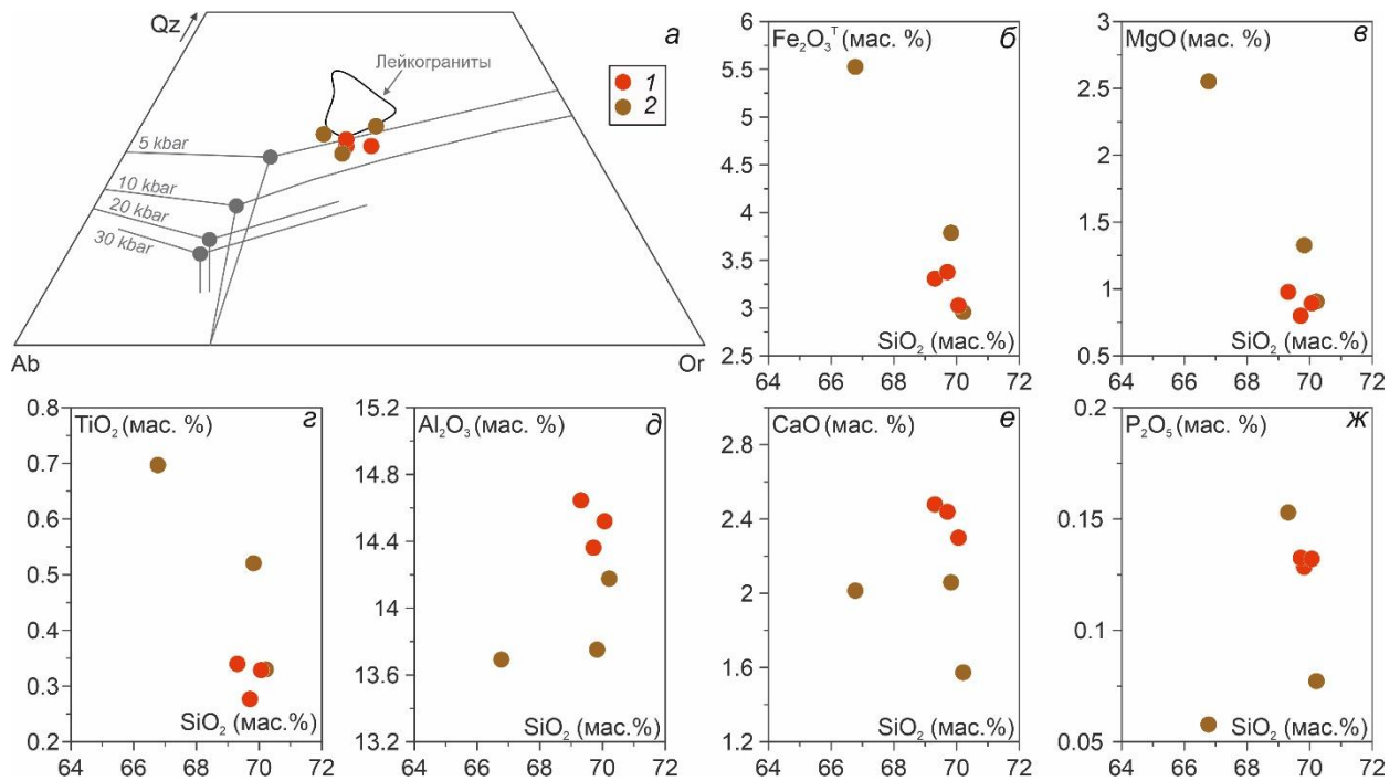
Рисунок 6.22. Особенности петрохимического состава гранитов комбинированных даек. а – диаграмма Qz-Ab-Or, круги и линии показывают точки эвтектики и котектические кривые для гаплогранитной системы при a_{\text{H}_2\text{O}} = 1 и различных давлениях (модифицировано Bartoli et al., 2016 по Holtz et al., 1992 ); б-ж – вариации содержаний петрогенных компонентов относительно \text{SiO}_2 (мас. %). 1 – биотит-роговообманковые граниты комбинированной дайки участка Тавыт-Даг; 2 – биотитовые граниты комбинированных даек участков Матут, Баянкол и РЛС. Черным контуром показаны лейкограниты комбинированных и простых даек (группа I).
