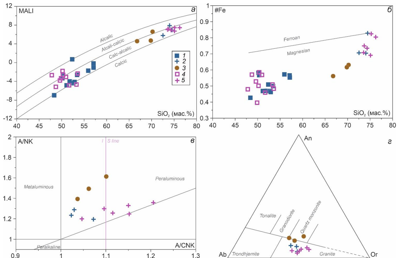
Рисунок 6.3. Классификационные диаграммы для пород комбинированных даек участков Баянкол, Матут и РЛС, а также простых базитовых и лейкогранитных даек. а – MALI - SiO_2 (Frost et al., 2001); б – FeO^{tot}/(FeO^{tot}+MgO) - SiO_2 (Frost et al., 2001); в – A/NK - A/CNK, I-S линия по (Chappell, White, 2001); з – Ab-An-Or, классификационные границы по (O'Connor, 1965). 1-3 – комбинированные дайки: 1 – габбро и диориты, 2 – лейкограниты, 3 – граниты; 4,5 – простые дайки: 4 – габбро и диориты, 5 – лейкограниты.
