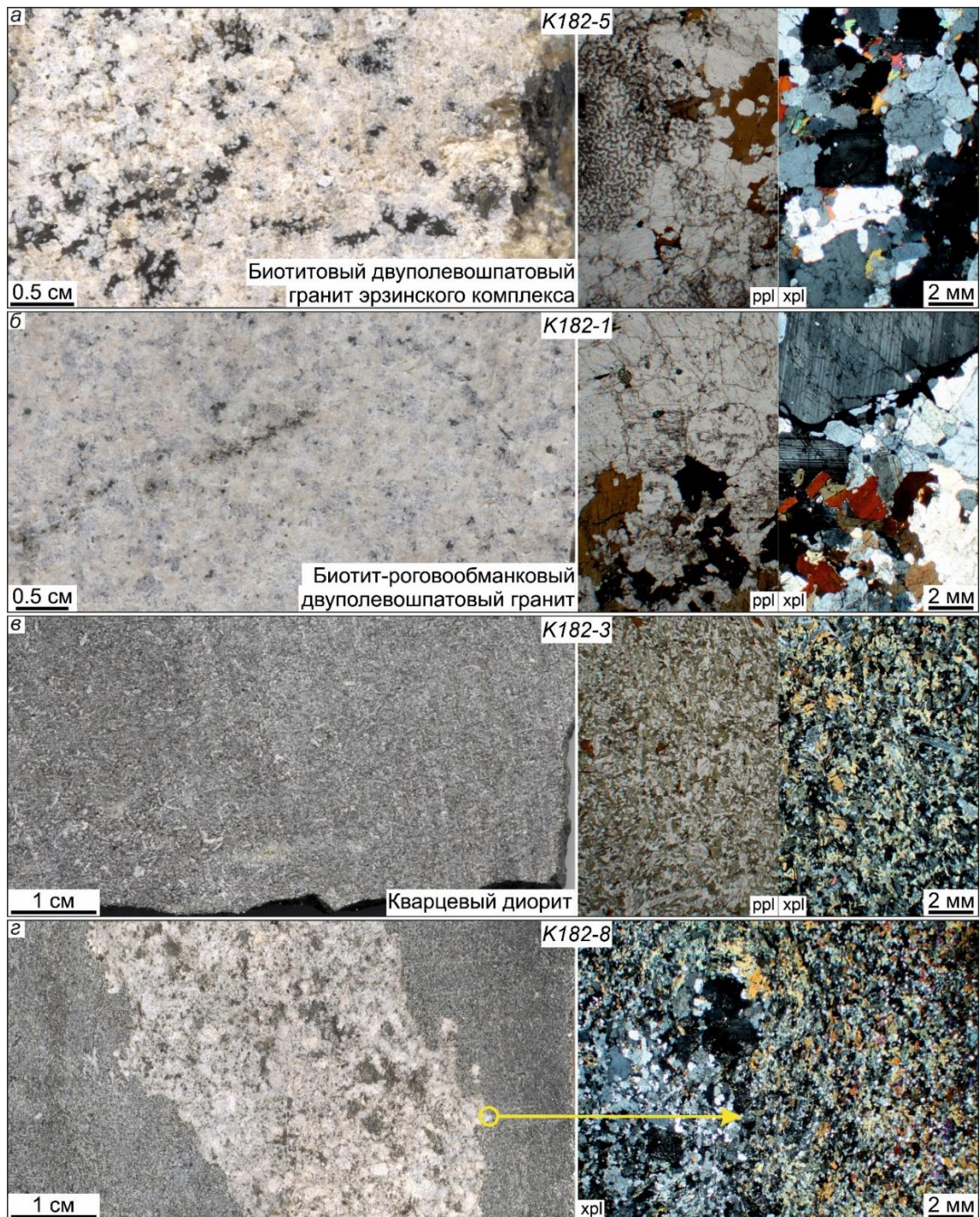
Рисунок 4.18. Петрография и взаимоотношения пород минглинг даек участка Восточный. г – четкий криволинейный контакт. В диоритах вблизи контакта наблюдается переориентировка темноцветных минералов и плагиоклаза, в гранитах – рекристаллизация кварца.
