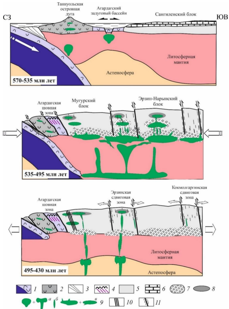
Рисунок 3.4. Реконструкция тектонической истории с отражением процессов базитового магматизма и сопряженного метаморфизма Сангиленского блока ранних каледонид на западной окраине Тувино-Монгольского континента по трем возрастным интервалам (Семенов, Полянский, 2023, с изменениями). 1 – океаническая кора и литосферная мантия; 2 – Таннуольская островная дуга; 3 – аккреционная призма; 4 – офиолиты Агардагской зоны; 5 – метаморфические комплексы коры Сангиленского блока – Grt-St-Ky сланцы (Ky-Sill типа); 6 – карбонаты чехла Сангиленского блока; 7–8 – ареалы высокоградиентного метаморфизма: 7 – УНТ гранулитовый метаморфизм в нижней/средней коре, 8 – гранулитовая зона НТ/LP метаморфизма в верхней коре (And-Sill типа); 9 – мантийные базитовые расплавы: а – области магмогенерации, б – магмоподводящие каналы, в – интрузивные камеры; 10 – дайки агардагского комплекса; 11 –разломы.
