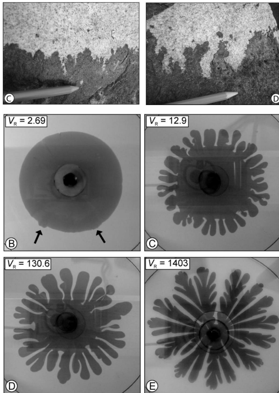
Рисунок 2.1. Типичное строение контактов контрастных по составу пород контрастных магматических систем (C, D) и результаты аналогового моделирования механического взаимодействия двух жидкостей с различным контрастом вязкости ( V_R ) (B-E) (Perugini, Poli, 2005).
