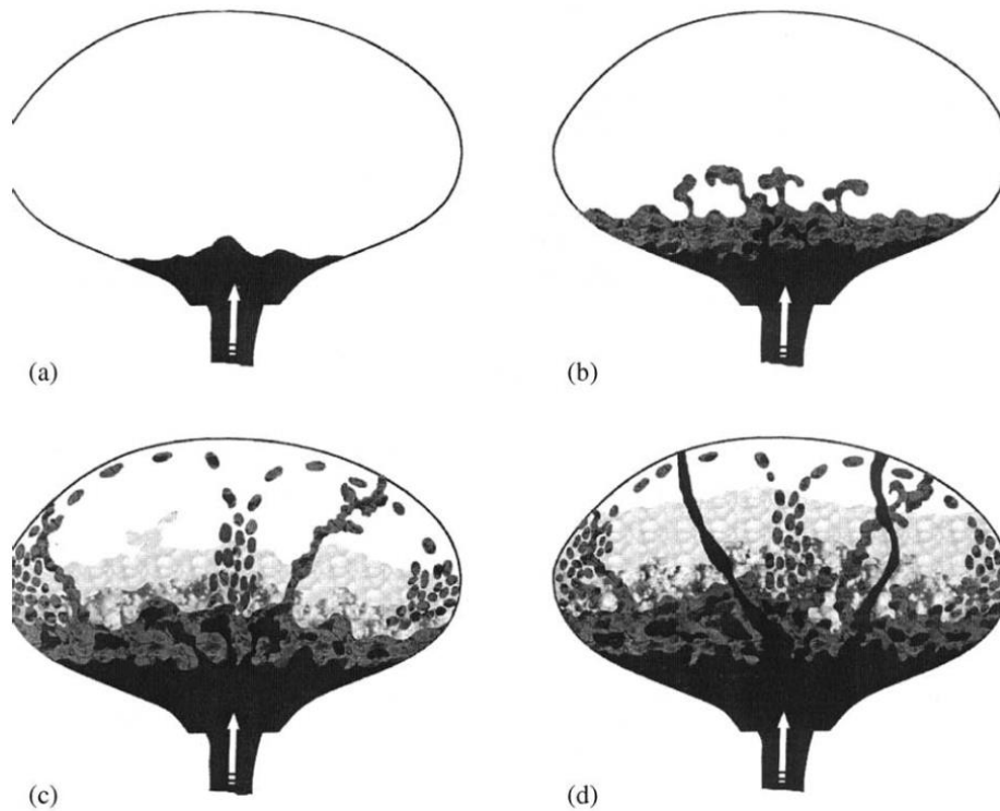
Рисунок 2.8. Обобщенная модель формирования ММЕ за счет образования промежуточного слоя гибридной магмы (Arvin et al., 2004): (a) внедрение мафической магмы в кислый магматический очаг; (b) взаимодействие между кислыми и мафическими магмами и развитие гибридной зоны; (c) продолжение смешения магм и развитие различных гибридных магматических зон. Дальнейшая конвекция приводит к рассеянию глобул гибридной магмы в верхние части магматического очага, где их слияние образует рои; (d) внедрение синплутонических даек на поздней стадии остывания магматического очага.
