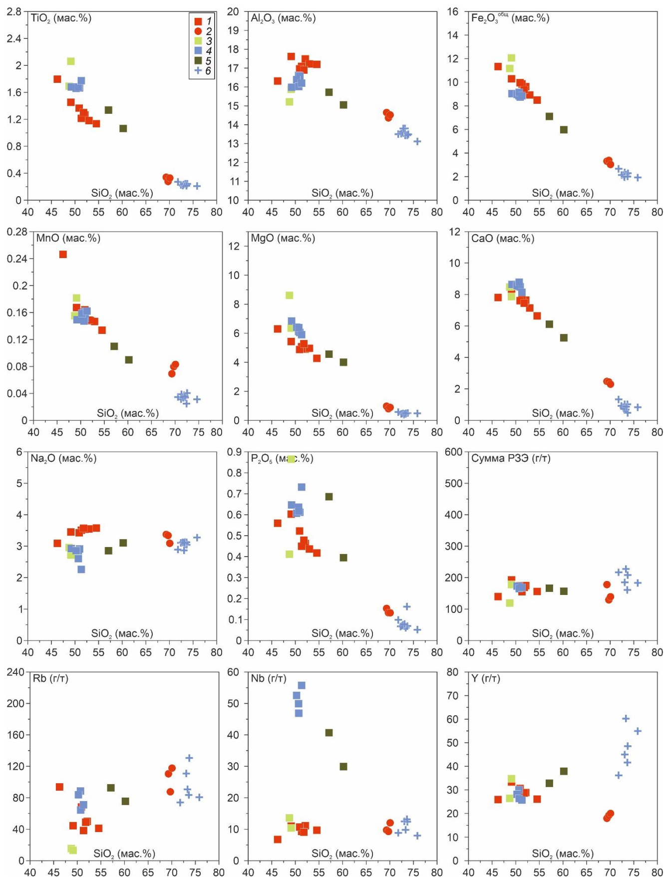
Рисунок 6.6. Содержания пороодообразующих (мас. %) и редких (г/т) элементов по отношению к \text{SiO}_2 для пород комбинированных даек участков Тавыт-Даг и Сайзырал. 1-2 – Тавыт-Даг: 1 – габбро и диориты, 2 – граниты; 3-6 – Сайзырал: 3 – габбро, 4 – диориты, 5 – породы переходных зон, 6 – лейкограниты.
