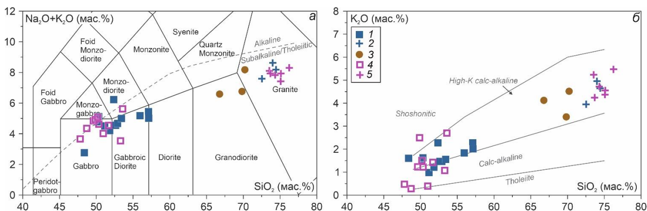
Рисунок 6.1. Классификационные диаграммы пород комбинированных даек участков Баянкол, Матут и РЛС, а также простых базитовых и лейкогранитных даек. а – \text{Na}_2\text{O}+\text{K}_2\text{O} - \text{SiO}_2 ( Middlemost, 1994 ); б – \text{K}_2\text{O} - \text{SiO}_2 ( Peccherilo, Taylor, 1976 ). 1-3 - комбинированные дайки: 1 – габбро и диориты, 2 – лейкограниты, 3 – граниты; 4,5 – простые дайки: 4 – габбро, 5 – лейкограниты.
