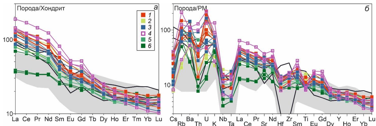
Рисунок 6.16. Обобщенные нормированные по хондриту кривые распределения редкоземельных элементов (а) и нормированные по примитивной мантии мультиэлементные диаграммы (б) для мафических пород комбинированных, синплутонических и простых даек. Данные для хондрита и примитивной мантии по (Sun, McDonough, 1989). 1 – дайка Тавыт-Даг, 2 – габбро дайки Сайзырал, 3 – дайки участков Матут, Баянкол, РЛС, 4 – простые дайки, 5 – дайки Стрелка, 6 – дайки Восточный. Серым полем показаны составы габброноритов Баянкольского массива, черным контуром – составы монцодиоритов Эрзинского массива по (Shelepaev et al., 2018).
