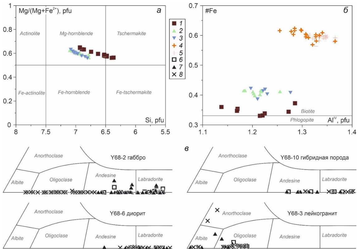
Рисунок 4.12. Классификационные диаграммы для амфиболов (а) (Leake et al., 1997), биотитов (б) (Deer et al., 2013) и полевых шпатов (в) пород комбинированной дайки Сайзырал. 1-5 – темноцветы: 1 – габбро, 2 – диоритов, 3 – гибридных пород, 4 – лейкогранитов (основная масса), 5 – лейкогранитов (гломероскопления). 6-8 – полевые шпаты: 6 – центральные части, 7 – промежуточные зоны, 8 – края.
