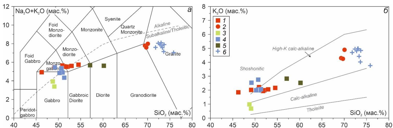
Рисунок 6.5. Классификационные диаграммы для пород комбинированных даек участков Тавыт-Даг и Сайзырал. а – \text{Na}_2\text{O}+\text{K}_2\text{O} - \text{SiO}_2 (Middlemost, 1994); б – \text{K}_2\text{O} - \text{SiO}_2 (Peccherillo, Taylor, 1976). 1-2 – Тавыт-Даг: 1 – габбро и диориты, 2 – граниты; 3-6 – Сайзырал: 3 – габбро, 4 – диориты, 5 – породы переходных зон, 6 – лейкограниты.
