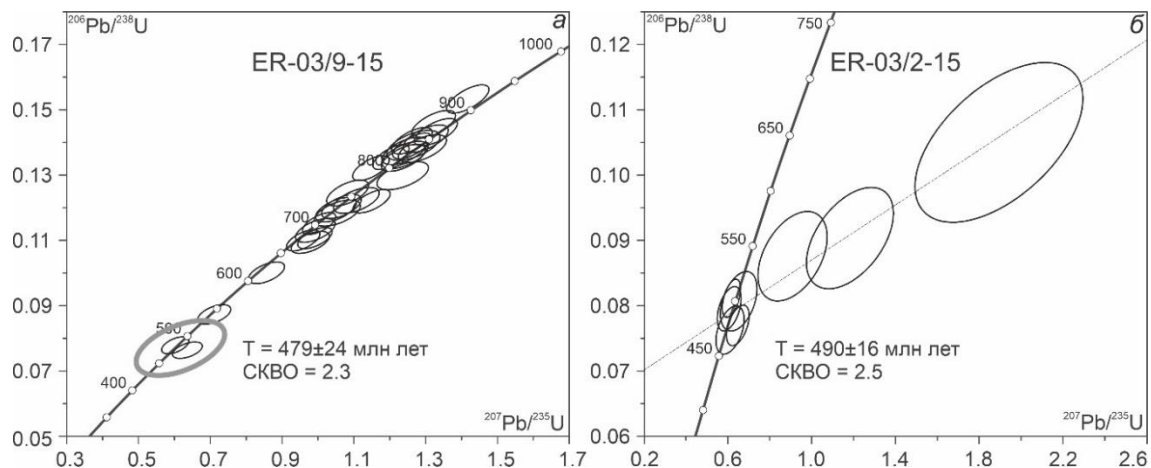
Рисунок 5.1. Диаграммы с конкордией для цирконов из гранитов (а) и диоритов (б) осевой зоны наиболее крупной комбинированной дайки участка Тавыт-Даг (Tsygankov et al., 2019).
