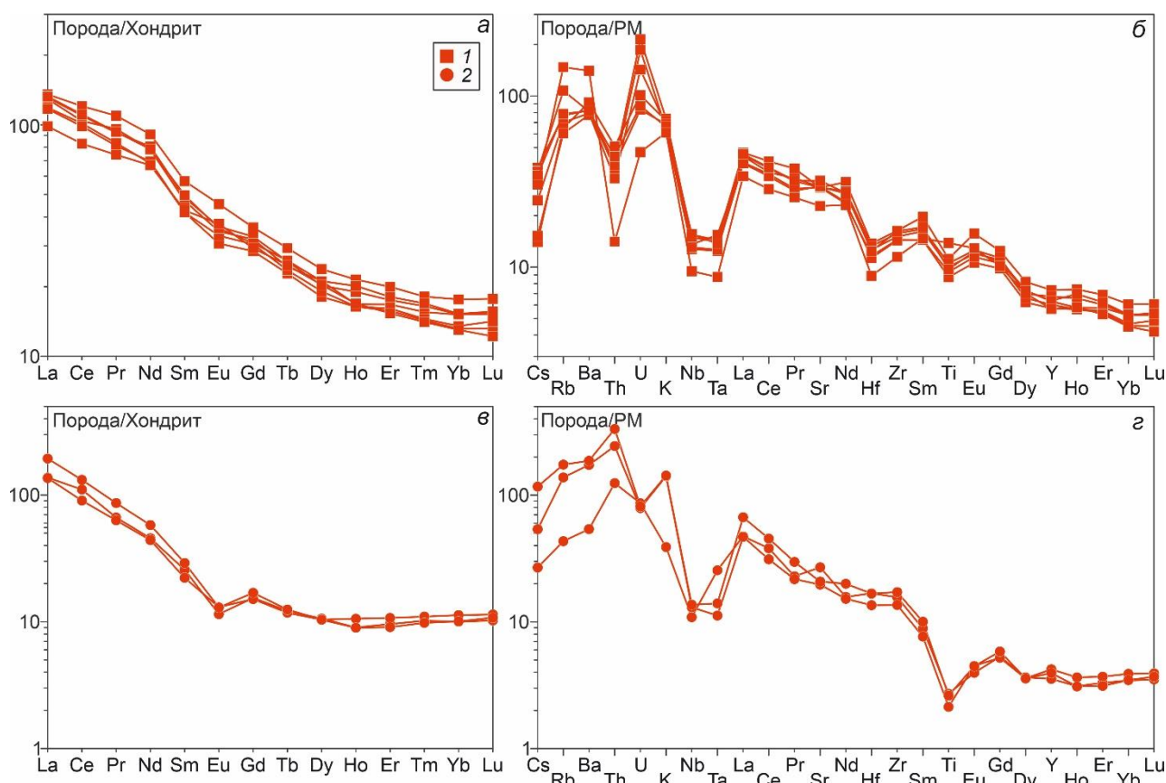
Рисунок 6.7. Нормированные по хондриту кривые распределения редкоземельных элементов (а, в) и нормированные по примитивной мантии мультиэлементные диаграммы (б, г) для пород комбинированных даек участка Тавыт-Даг. Данные для хондрита, примитивной мантии, MORB и OIB по (Sun, McDonough, 1989). 1 – габбро и диориты, 2 – граниты.
