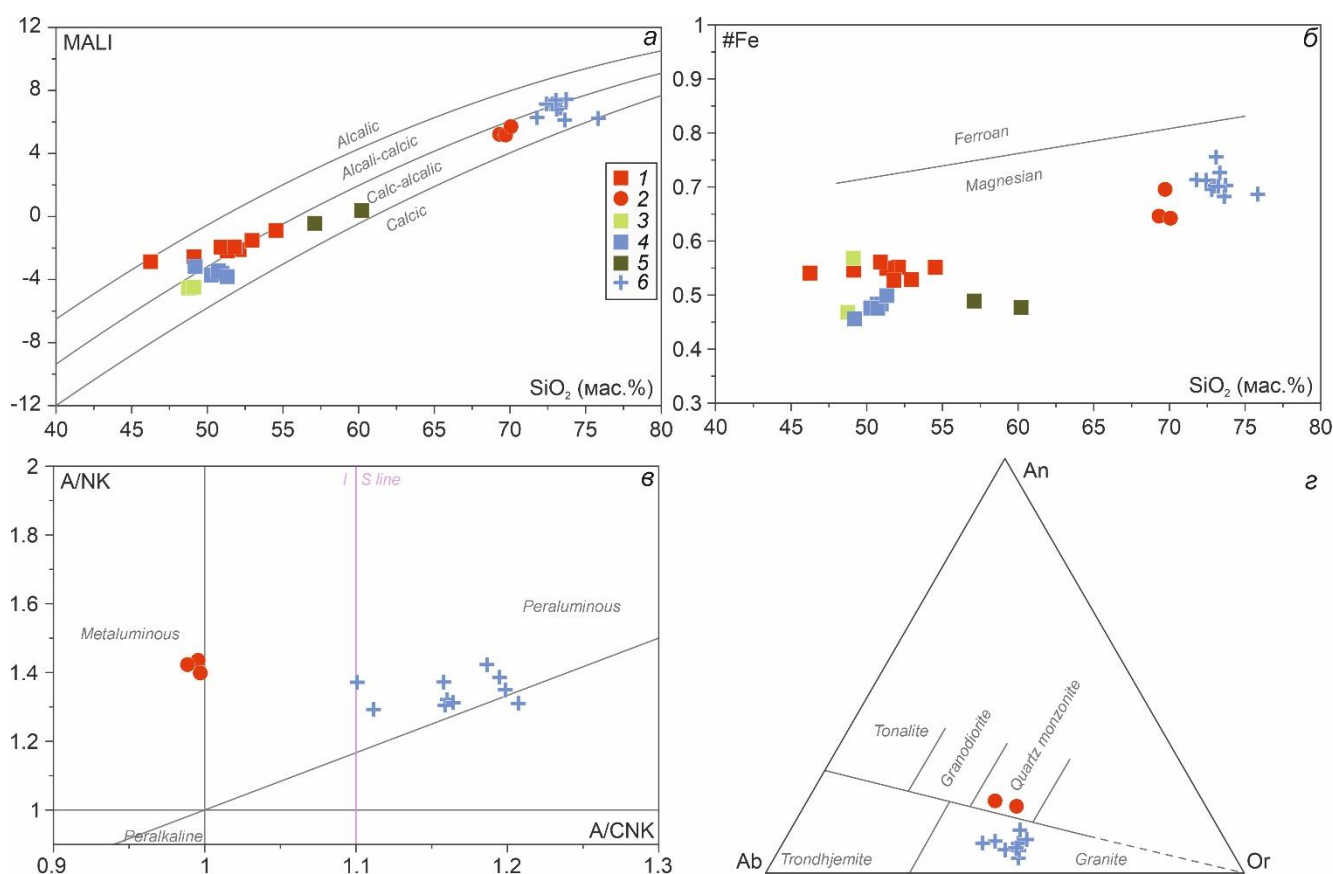
Рисунок 6.8. Классификационные диаграммы для пород комбинированных даек участков Тавыт-Даг и Сайзырал. а – MALI - SiO_2 (Frost et al., 2001); б – FeO^{tot}/(FeO^{tot}+MgO) - SiO_2 (Frost et al., 2001); в – A/NK - A/CNK, I-S линия по (Chappell, White, 2001); г – Ab-An-Or, классификационные границы по (O'Connor, 1965). 1-2 – Тавыт-Даг: 1 – габбро и диориты, 2 – граниты; 3-6 – Сайзырал: 3 – габбро; 4 – диориты; 5 – породы переходных зон; 6 – лейкограниты.
