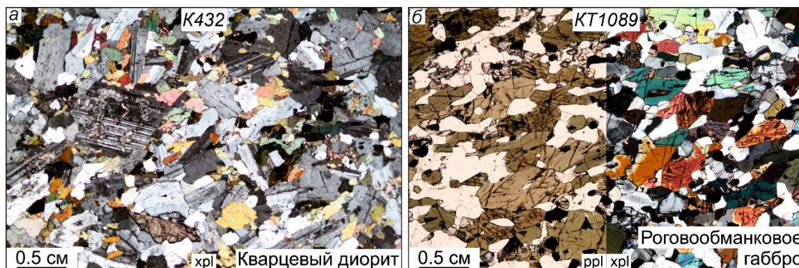
Рисунок 4.5. Петрографическая характеристика мафических пород комбинированных даек участков Баянкол, Матут, РЛС.
