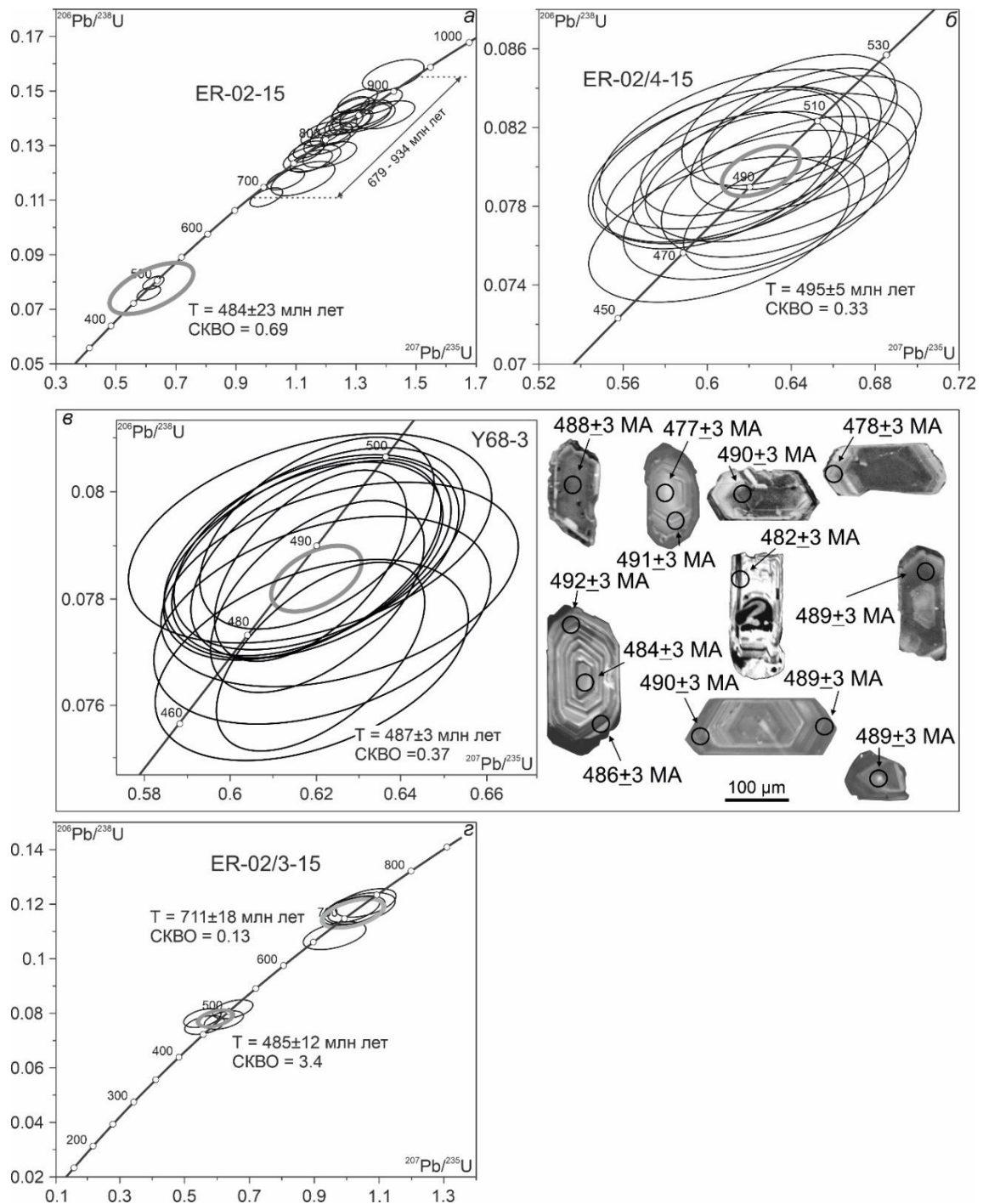
Рисунок 5.2. Диаграммы с конкордией и катодоллюминесцентные изображения цирконов из пород участка Сайзырал: а – вмещающие гнейсограниты эрзинского комплекса; б – лейкогранит из средней части дайки; в – лейкогранит из верхней части дайки (Yakovlev et al., 2024); г – диорит из нижней части дайки. Пробы с индексом ER по (Tsygankov et al., 2019).
