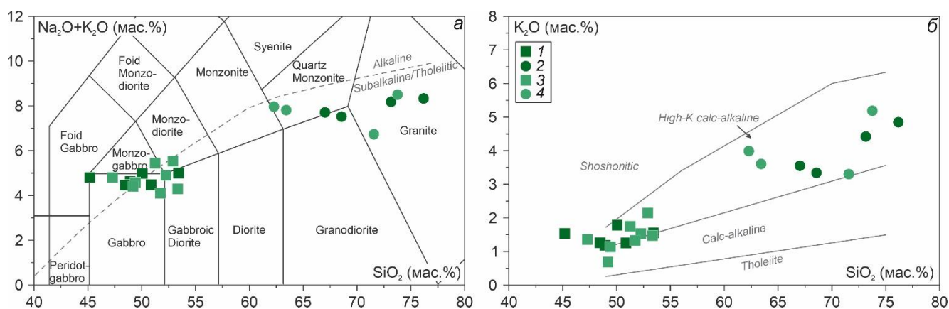
Рисунок 6.10. Классификационные диаграммы для пород синплутонических даек участков Стрелка и Восточный. а – \text{Na}_2\text{O}+\text{K}_2\text{O} - \text{SiO}_2 (Middlemost, 1994); б – \text{K}_2\text{O} - \text{SiO}_2 (Peccherillo, Taylor, 1976). 1,2 – Восточный: 1 – габбро и диориты, 2 – гранитоиды; 3,4 – Стрелка: 3 – габбро и диориты, 4 – гранитоиды
