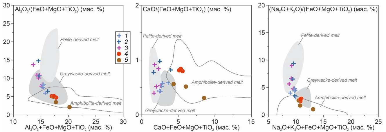
Рисунок 6.20. Диаграммы составов экспериментальных расплавов, полученных в результате дегидратационного плавления метаосадочных пород и амфиболитов (Patiño Douce, 1999; Rollinson, 2015), а также составы изученных образцов гранитоидов комбинированных даек. 1-3 – лейкограниты (группа I): 1 – участок Сайзырал; 2 – участки Матут, Баянкол, РЛС; 3 – простые дайки; 4, 5 – граниты (группа II): 4 – участок Тавыт-Даг, 5 – участки Матут, Баянкол и РЛС.
