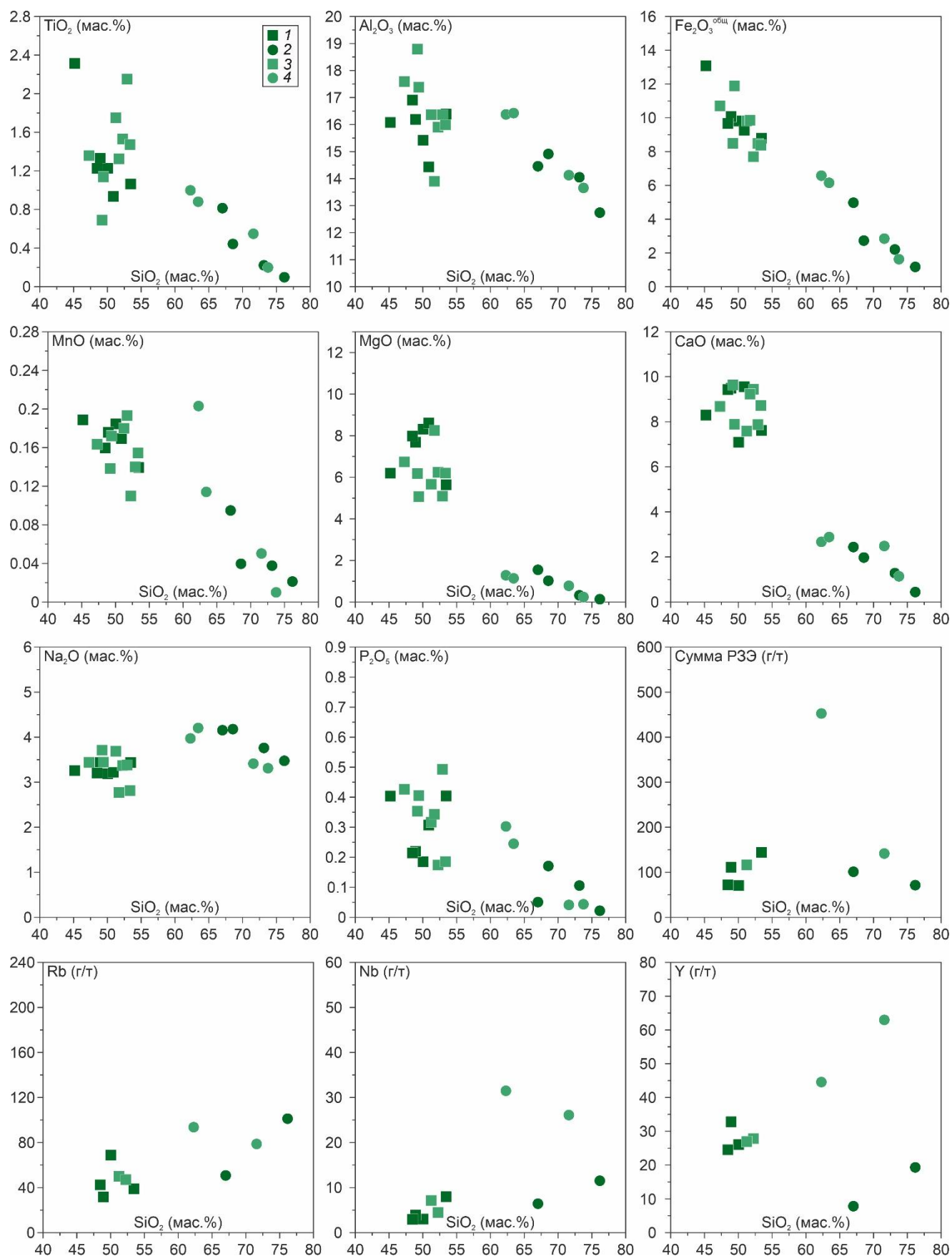
Рисунок 6.11. Содержания породообразующих (мас. %) и редких (г/т) элементов по отношению к \text{SiO}_2 для пород синплутонических даек участков Стрелка и Восточный. 1,2 – Восточный: 1 – габбро и диориты, 2 – гранитоиды; 3,4 – Стрелка: 3 – габбро и диориты, 4 – гранитоиды.
