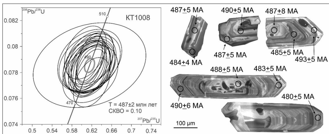
Рисунок 5.4. Диаграммы с конкордией и катодоллюминесцентные изображения цирконов из порфировидных кварцевых сиенитов Нижнеэрзинского массива, участок Стрелка (Кармышева и др., 2022а).
