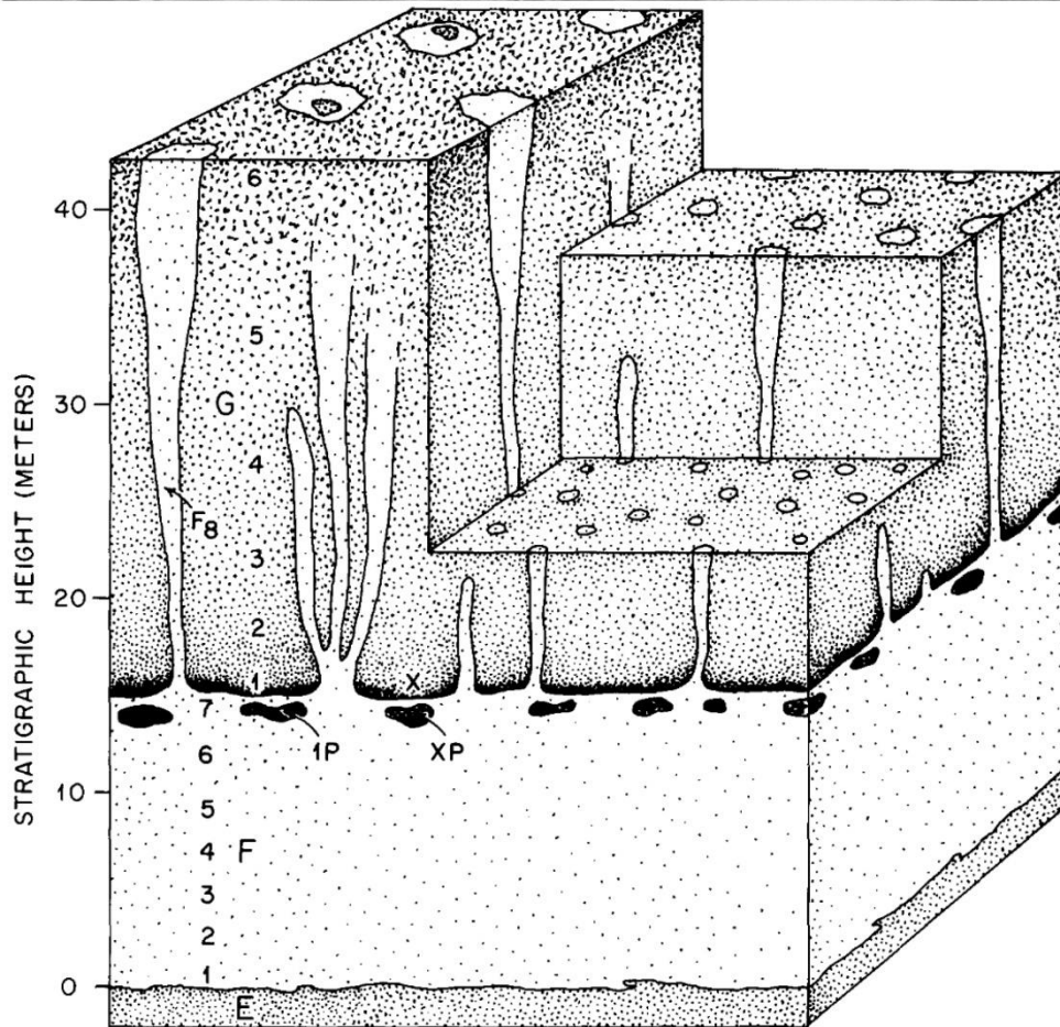
Рисунок 2.5. Вид на обнажение и модельное строение габбро-диоритовых интрамагматических лавовых потоков (расслоенных интрузий) ( Chapman, Rhodes, 1992 ).
