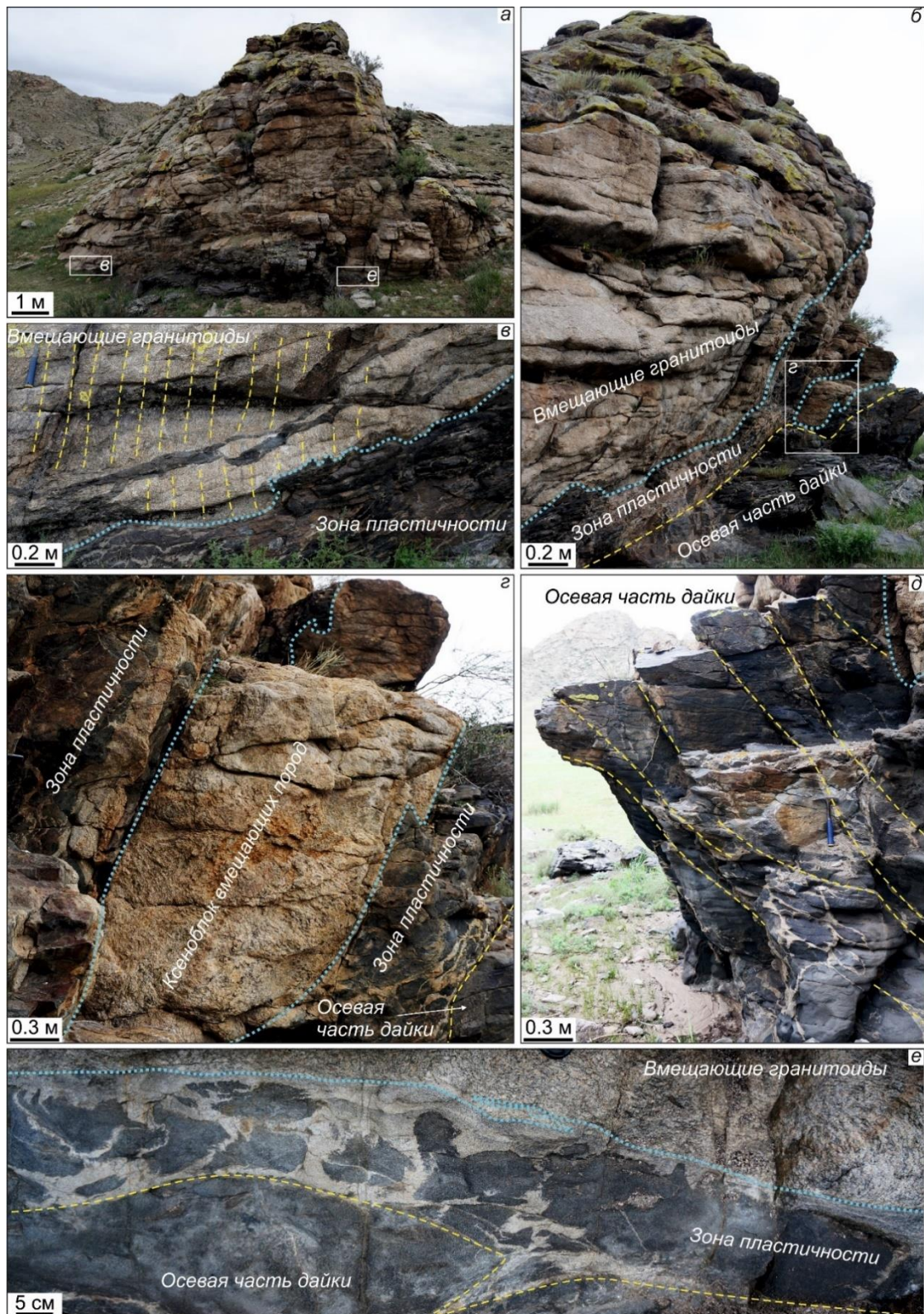
Рисунок 4.6. Внутреннее строение комбинированных даек участка Тавыт-Даг. а – общий вид на обнажение; б – западная сторона обнажения; в – эшелонированная система базитовых даек, ответвляющихся от наиболее мощной минглинг дайки; г – ксеноблок вмещающих гранитоидов Матутского массива; д – восточная сторона обнажения, гранитоидные «жилы» формируют сетчатую структуру осевой части дайки; е – характерные черты зоны пластичности наиболее мощной дайки. Желтым пунктиром показана магматическая полосчатость вмещающих пород, ориентировка гранитоидных «жил» в осевой части дайки, а также граница зоны пластичности и осевой части дайки. Голубым пунктиром показан контакт комбинированной дайки с вмещающими породами, а также ориентировка гранитоидных «жил» в осевой части дайки.
