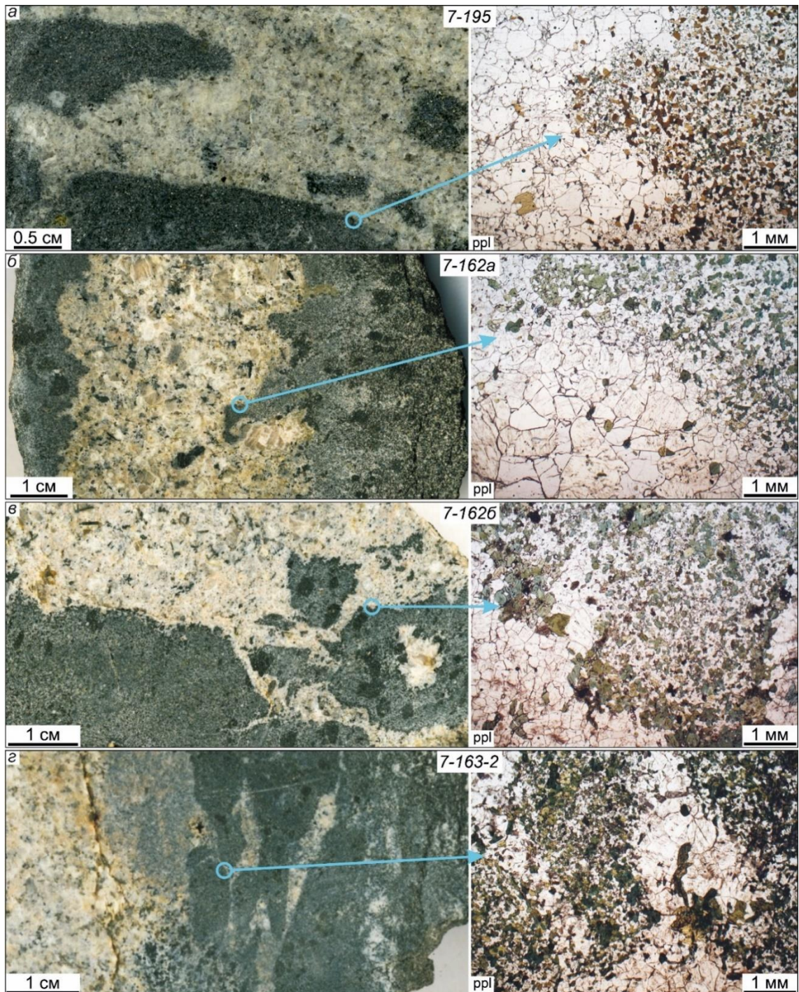
Рисунок 4.15. Взаимоотношения контрастных пород синплутонических даек участка Стрелка. а – четкий криволинейный контакт; б – пламенивидные и микрофестончатые контакты; в – рваный контакт, вблизи которого в базитах повышается концентрация и размер зерен амфибола и биотита; з – сложное строение контактовой зоны.
