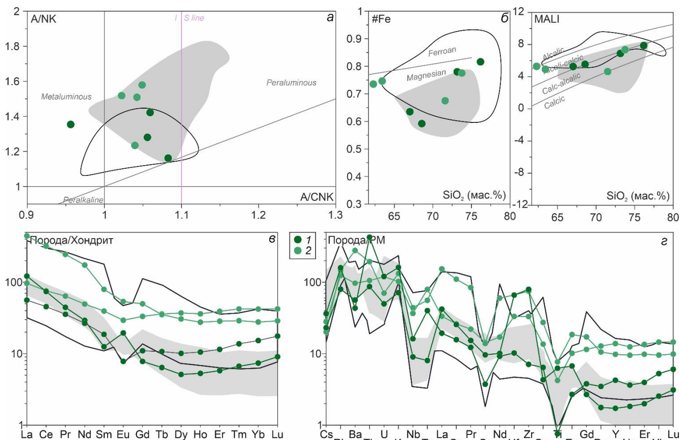
Рисунок 6.23. Особенности вещественного состава гранитоидов синплутонических даек. a – A/NK - A/CNK, I-S линия по (Chappell, White, 2001); б – \text{FeO}^{\text{tot}}/(\text{FeO}^{\text{tot}}+\text{MgO}) - \text{SiO}_2 (Frost et al., 2001); в – нормированные по хондриту кривые распределения редкоземельных элементов; г – нормированные по примитивной мантии мультиэлементные диаграммы (Sun, McDonough, 1989). 1 – участок Восточный; 2 – участок Стрелка. Черным контуром показаны гранитоиды ухадагского комплекса (Кармышева и др., 2022а), серым полем – параавтохтонные граниты эрзинского мигматит-гранитного комплекса (Кармышева и др., 2017).
