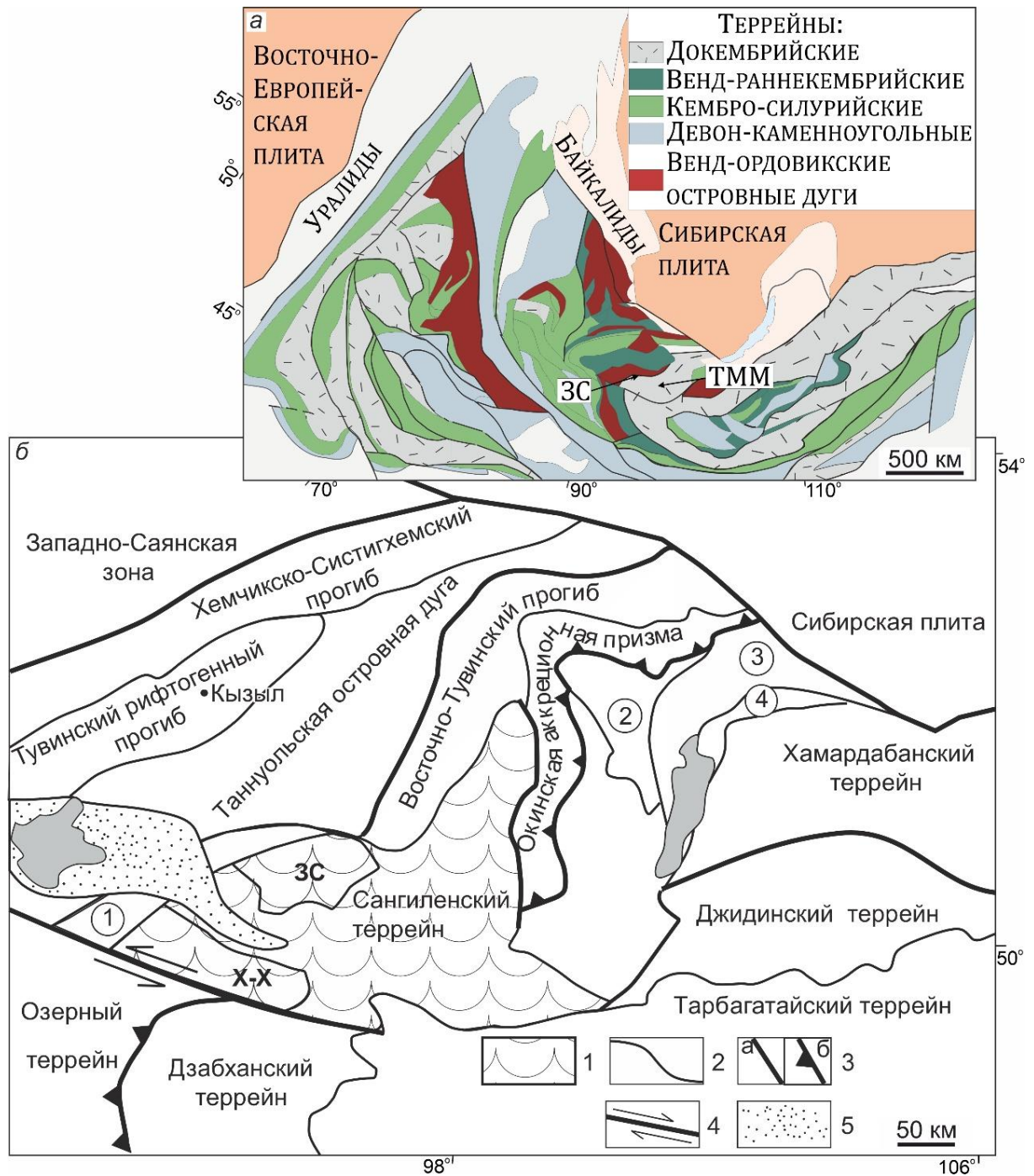
Рисунок 3.1. Положение Тувино-Монгольского массива в структурах ЦАСП. а – упрощенная тектоническая схема ЦАСП по (Lehmann et al., 2010, составлена на основе Sengor et al., 1993; Xiao et al., 2008). ТММ – Тувино-Монгольский микроконтинент, ЗС – Западный Сангилен; б – Структурно-тектоническая схема Северной Монголии и примыкающей части Алтае-Саянской области по (Полянский и др., 2023, составлена на основе Кузьмичев, 2004; Монгуш, 2012; Ярмолук, Дегтярев, 2019). 1 – Сангиленский террейн (показаны блоки Западный Сангилен (ЗС) и Хан-Хухей (Х-Х)); 2 – границы между структурными элементами; 3 – разломы неопределенной кинематики (а), надвиги (б); 4 – сдвиги; 5 – кайнозойские осадочные породы. Цифры в кружках – террейны: 1 – Агардагский, 2 – Дархатский, 3 – Гарганский, 4 – Ильчирский.
