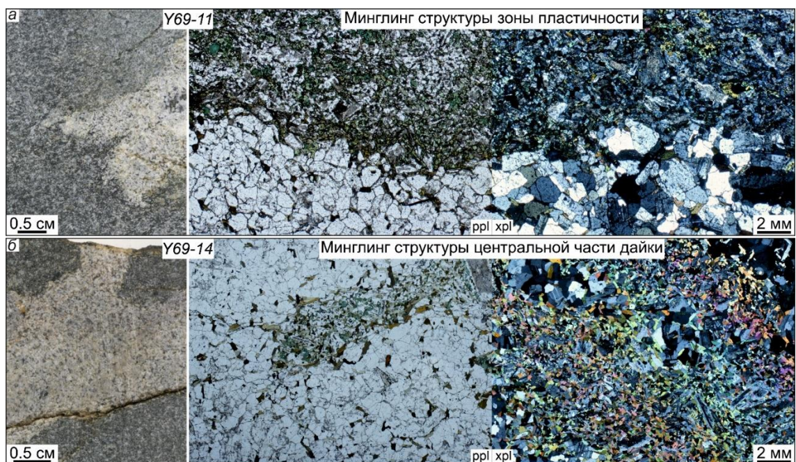
Рисунок 4.8. Взаимоотношения контрастных пород комбинированных даек участка Тавыт-Даг.
