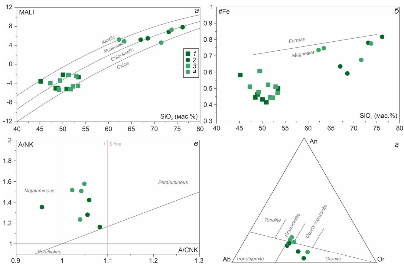
Рисунок 6.12. Классификационные диаграммы для пород синплутонических даек участков Стрелка и Восточный. a – MALI - \text{SiO}_2 (Frost et al., 2001); б – \text{FeO}^{\text{tot}}/(\text{FeO}^{\text{tot}}+\text{MgO}) - \text{SiO}_2 (Frost et al., 2001); в – A/NK - A/CNK, I-S линия по (Chappell, White, 2001); г – Ab-An-Or, классификационные границы по (O'Connor, 1965). 1,2 – Восточный: 1 – габбро и диориты, 2 – гранитоиды; 3,4 – Стрелка: 3 – габбро и диориты, 4 – гранитоиды.
