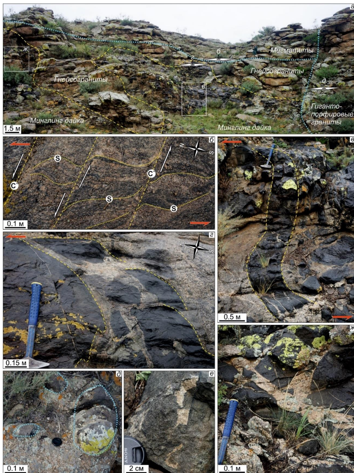
Рисунок 4.17. Строение синплутонических даек участка Восточный. а – общий вид обнажения; б – индикаторные деформационные структуры, план; в , г – S-образные вязко-пластичные деформационные структуры, косое сечение; д – мафические включения в гигантопорфировых гранитах, план; е – поздняя базитовая дайка; ж – минглинг дайка второй генерации. Голубым пунктиром показан контакт мигматитов и гнейсогранитов эрзинского комплекса, мафических включений и гигантопорфировых гранитов. Желтым пунктиром показан контакт гнейсогранитов и минглинг даек, а также индикаторные деформационные структуры.
