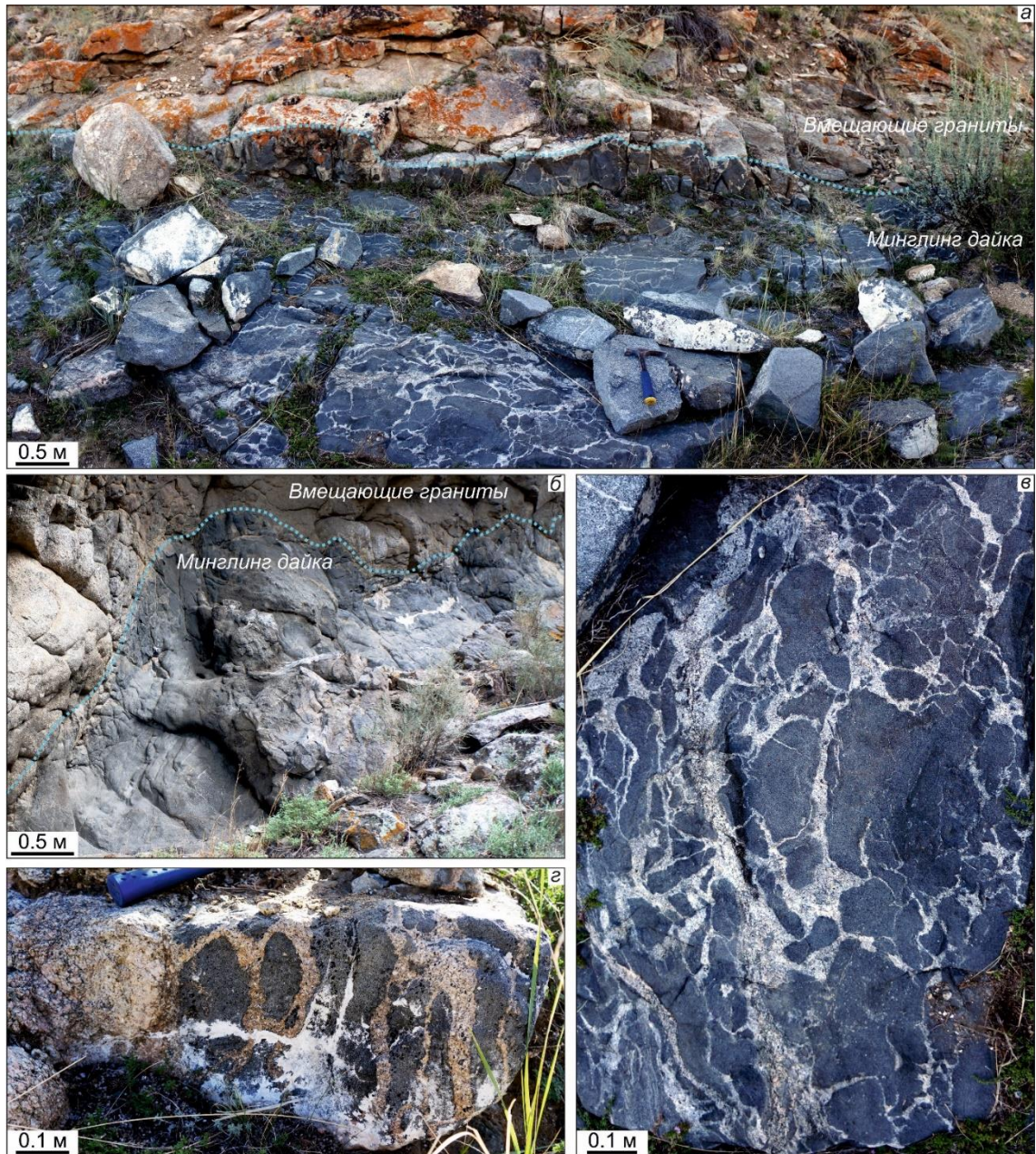
Рисунок 4.13. Внутреннее строение синплутонических даек участка Стрелка. а – общий вид наиболее представительного обнажения; б – субвертикальный контакт преимущественно базитовой дайки и граносиенитов Нижнеэрзинского массива; в – сетчатая структура, план; г – сетчатая структура, вертикальный срез. Голубым пунктиром показаны контакты даек и гранитоидов Нижнеэрзинского массива.
