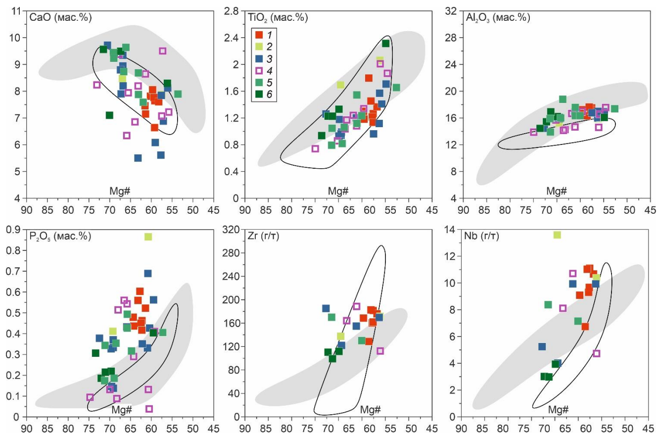
Рисунок 6.14. Вариации содержания петрогенных (мас. %) и редких (г/т) элементов в мафических породах комбинированных, синплутонических и простых даек относительно \text{Mg\#} . 1 – дайка Тавыт-Даг, 2 – габбро дайки Сайзырал, 3 – дайки участков Матут, Баянкол, РЛС, 4 – простые дайки, 5 – дайки Стрелка, 6 – дайки Восточный. Серым полем показаны составы габброноритов, черным контуром – составы монцодиоритов Баянкольского и Эрзинского массивов (Shelepaev et al., 2018).
