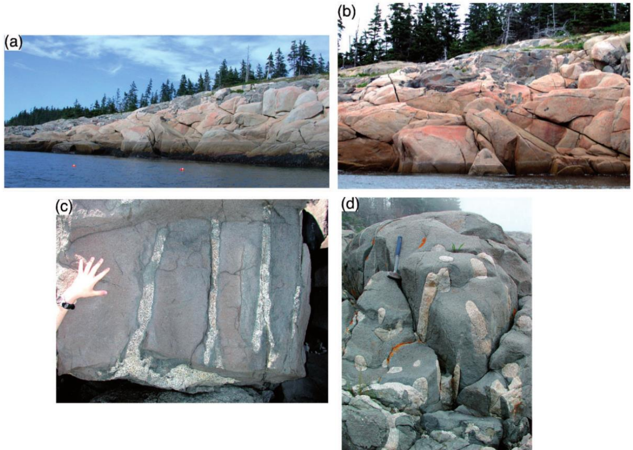
Рисунок 2.6. Внутреннее строение габбро-гранитных интрамагматических лавовых потоков (расслоенных интрузий) ( Wiebe, Hawkins, 2015 ).
