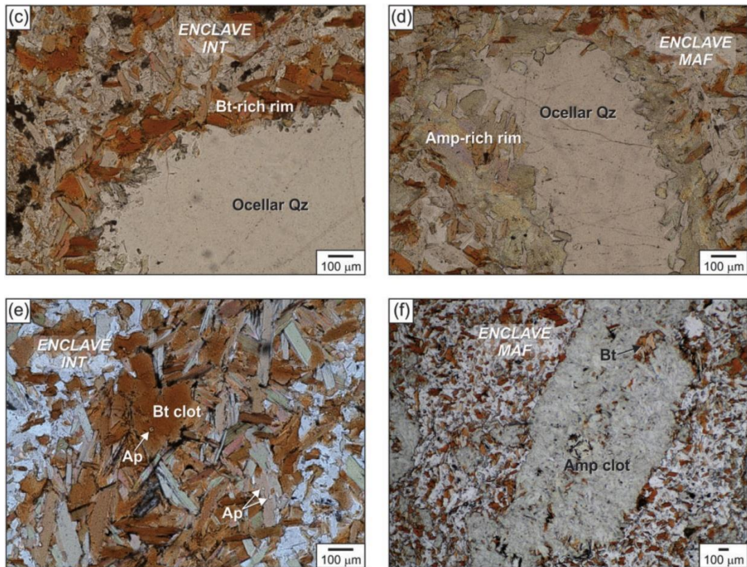
Рисунок 2.2. Примеры неравновесных петрографических структур в гибридных породах, формирующихся при взаимодействии контрастных по составу магм. c, d – кварцевые «глазки» с биотитовой ( c ) и амфиболовой оторочкой ( d ); e, f – биотитовые ( e ) и амфиболовые ( f ) гломероскопления (Ubidé et al., 2014).
