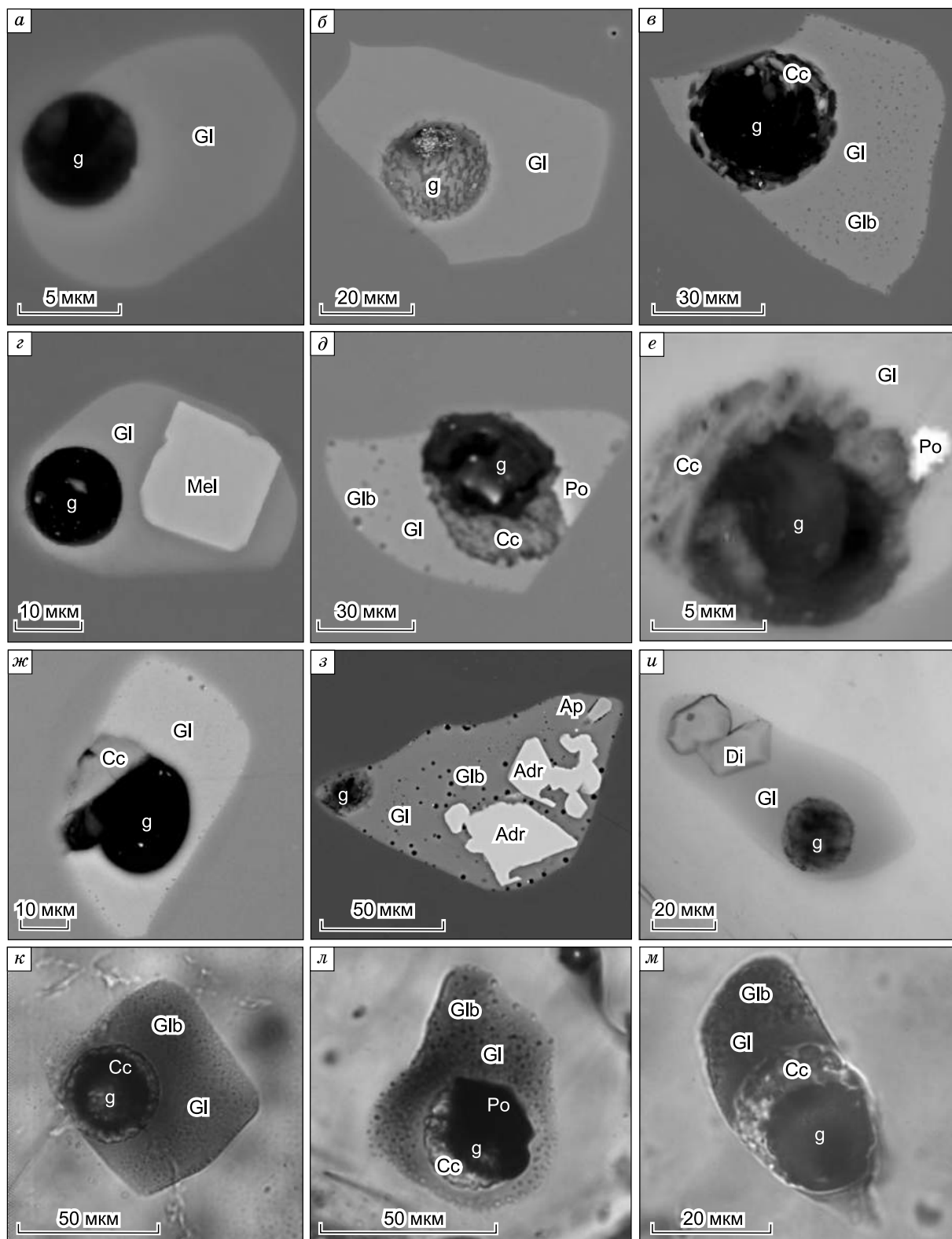
Рис. 5. Включения расплава в нефелине из ксенолита OL-006-05:
