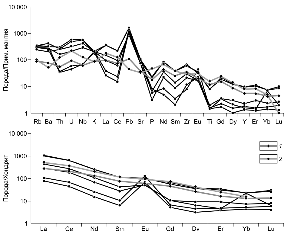
Рис 12. Спектры распределения несовместимых и редкоземельных элементов для оливин-слюда-ных ийолитов обр. OL-006-05 и OL-264с (1) и стеклов расплавных включений в нефелине из обр. OL-006-05 (2).
