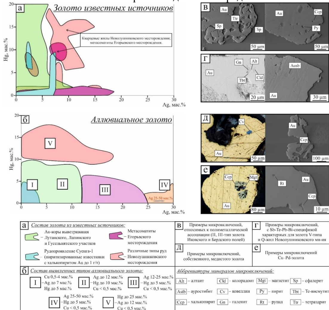
Рис.7. Иллюстрация комплексная. Поля составов золота аллювиальных россыпей и известных коренных источников, примеры микровключений.
