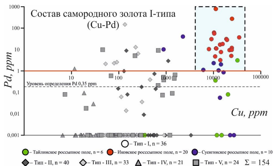
Рис.5. Микропримесный состав золота, отношения содержаний Pd к Cu.
