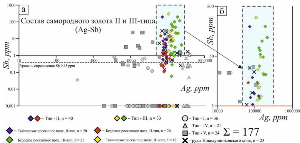
Рис.6. Микропримесный состав золота, отношения содержания Sb к Ag.
